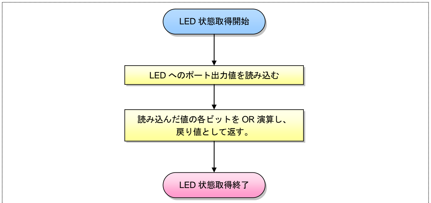
図 8.2-43 LED 点灯／消灯状態参照のフローチャート
