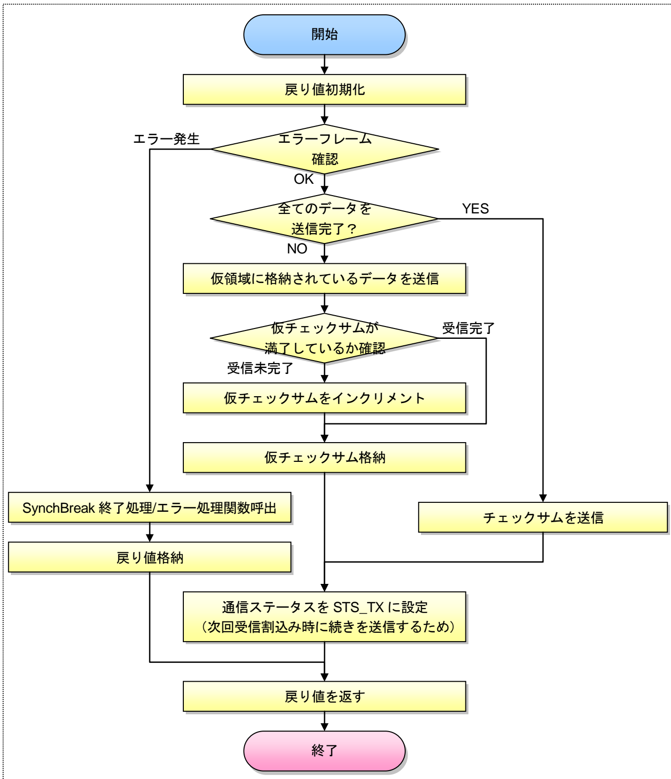
図 10.2-23. UART データ送信処理 sts_tx フローチャート
