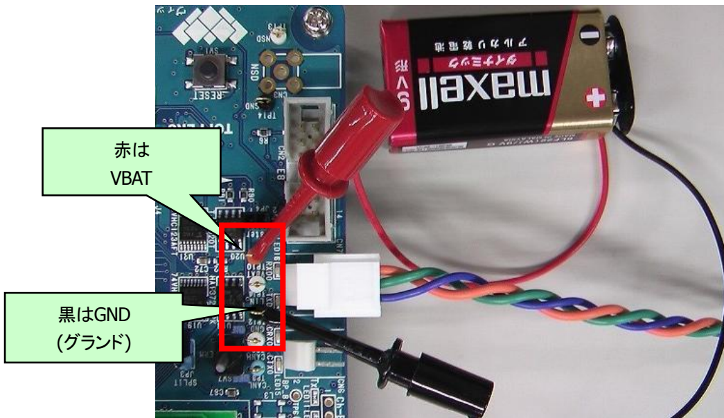
図 10.4-5 LIN デバイスドライバ動作確認手順 5
