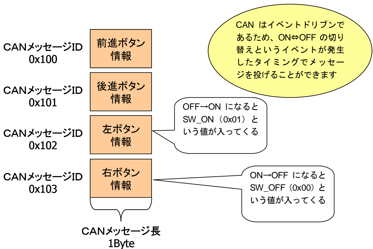
図 11.1-2 CAN メッセージ概要図
