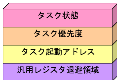
図 3.4-3 TCB 構造の例
