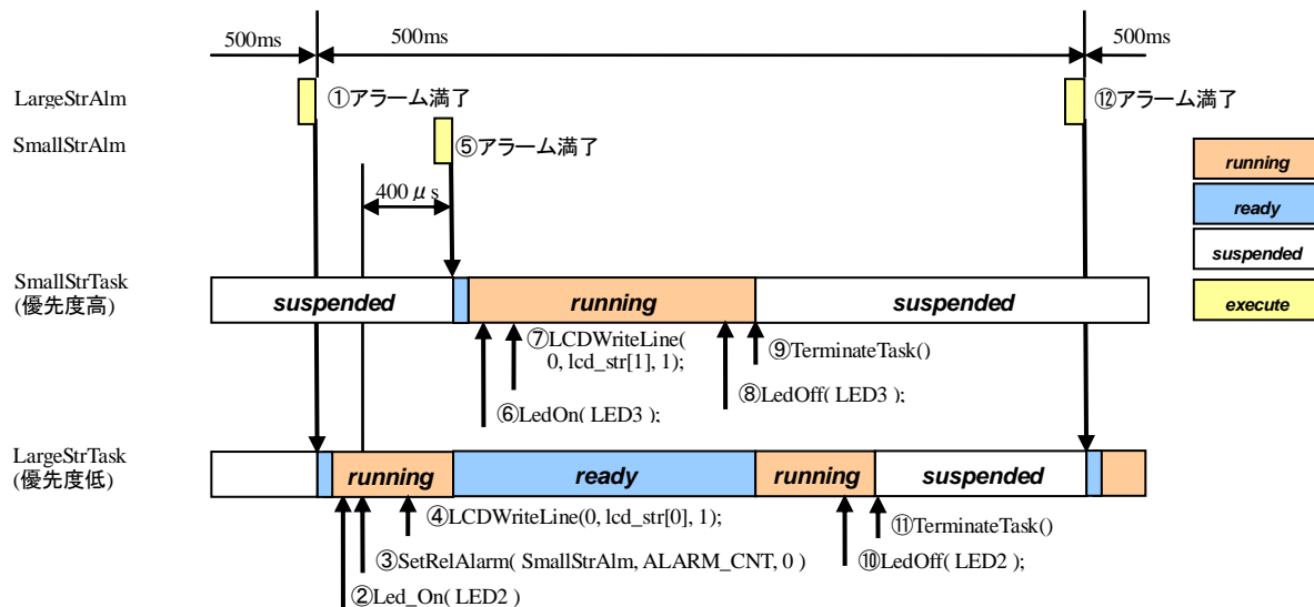
図 12.2-1 リソース未使用プログラムの動作
