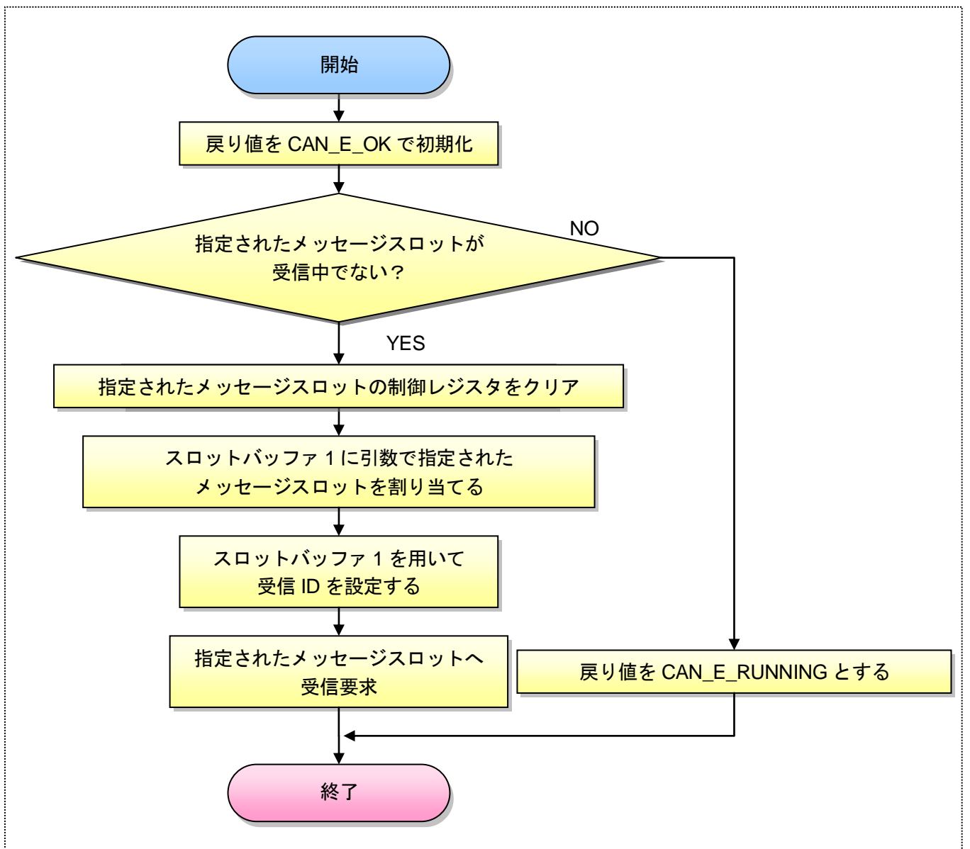
図 9.2-6 CAN 受信設定依存部関数 hw_can_set_rec フローチャート
