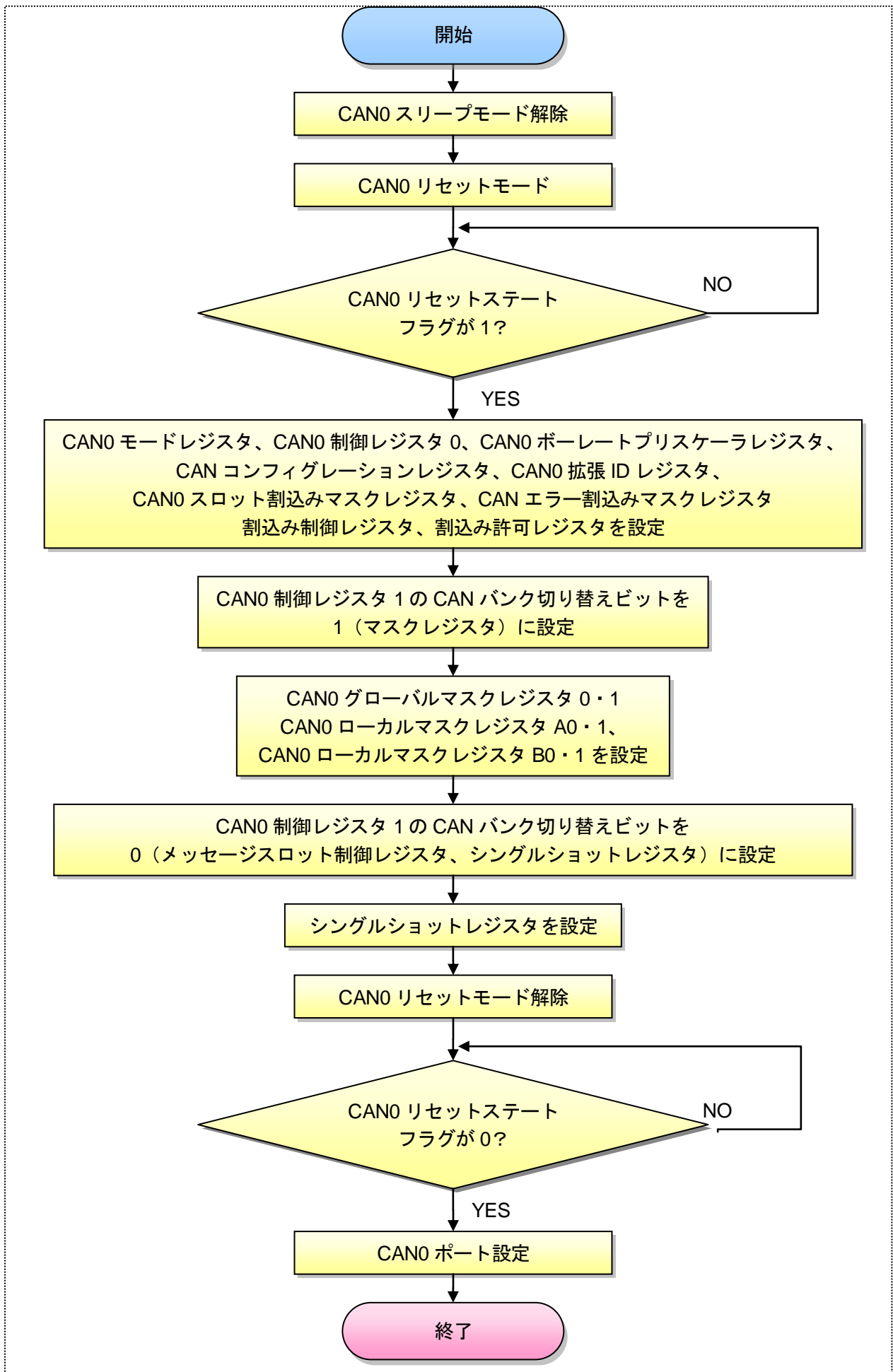
図 9.2-4 CAN 初期化依存部関数 hw_can_init フローチャート
