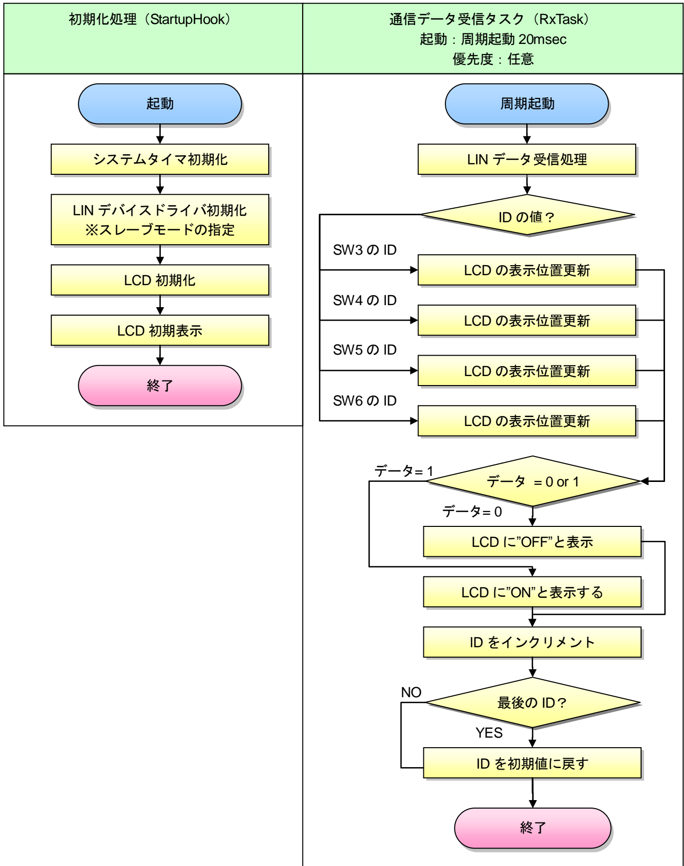
図 10.3-8 LIN デバイスドライバ動作確認アプリ仕様
