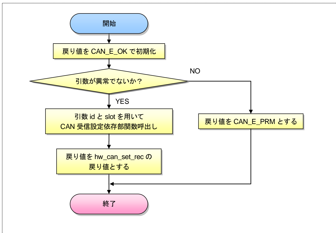
図 9.2-10 CAN 受信設定 API CanSetRec フローチャート
