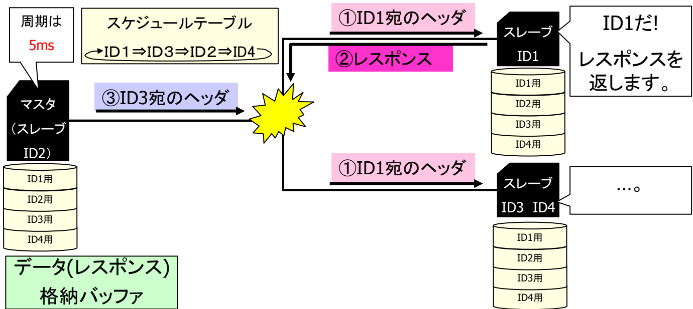
図 10.1-11 LIN 通信 異常パターン
