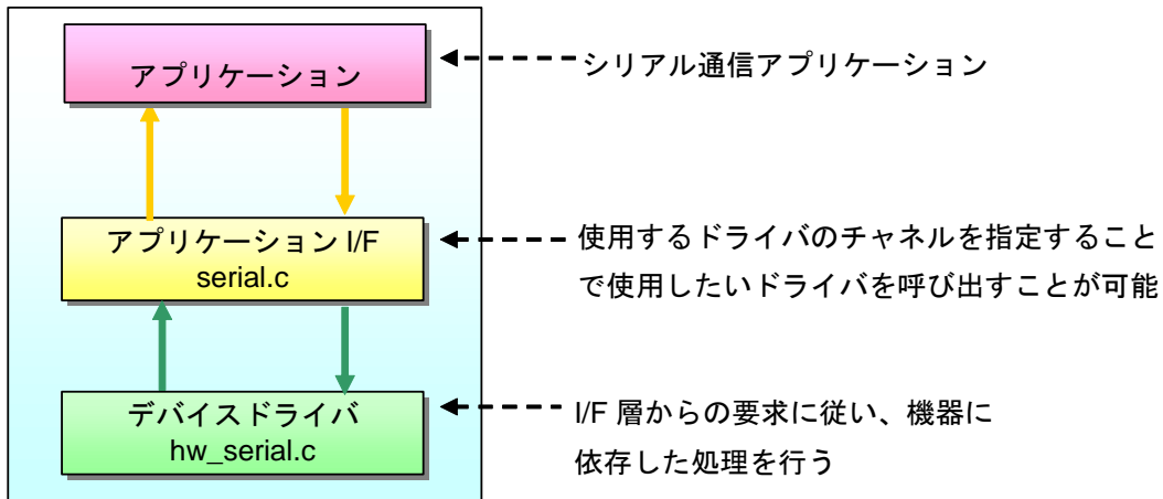
図 8.2-6 シリアルドライバの階層構造例
