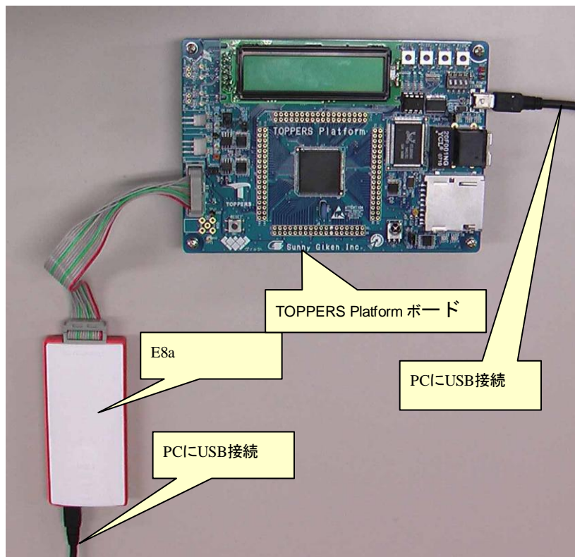
図 5.3-1 TOPPERS Platform ボード開発環境接続
