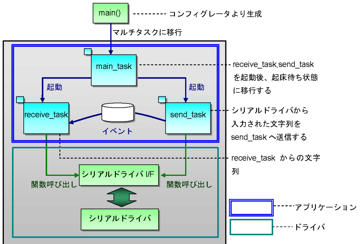
図 8.2-50 タスク構成図
