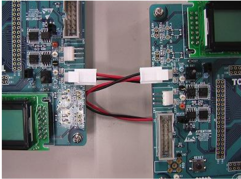
図 9.3-6 CAN ケーブル接続
