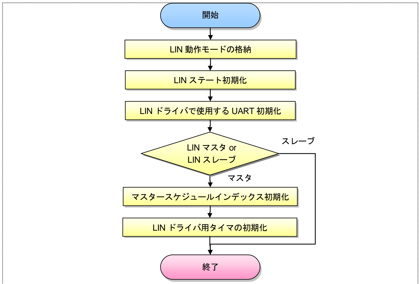
図 10.2-25. LIN マスタの初期化 API LinInit フローチャート
