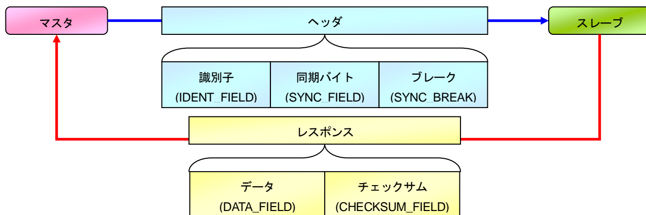
図 10.1-4 ノード間の通信
