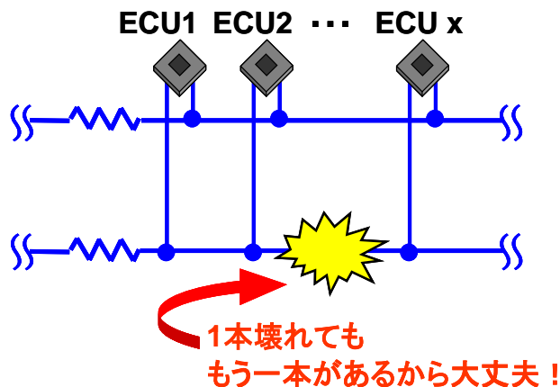
図 9.1-2 High Speed CAN と Low Speed CAN
