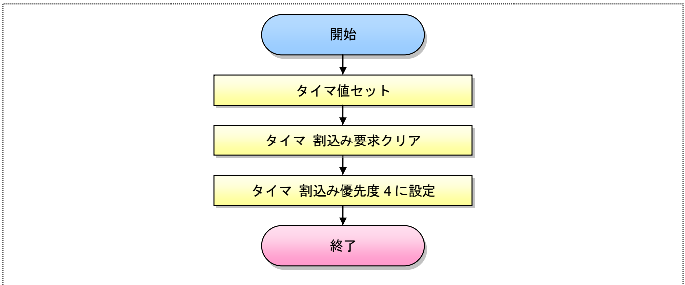
図 10.2-11. タイマ設定依存部関数 hw_lin_timer_set フローチャート
