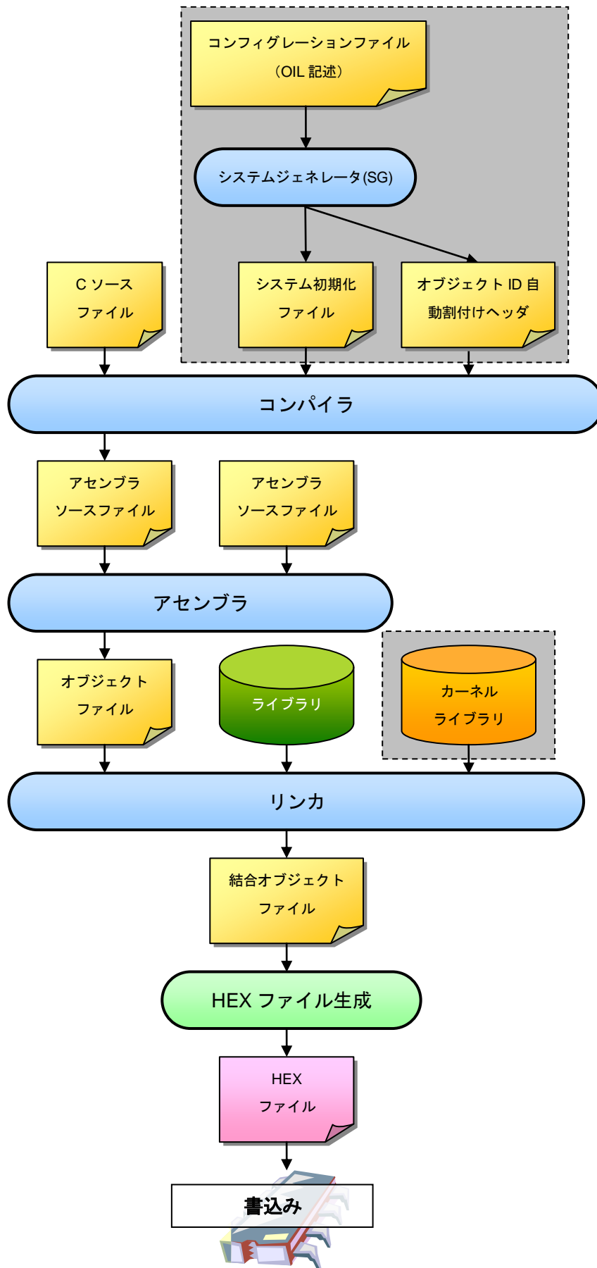
図 4.2-2 TOPPERS Automotive Kernel 使用時の HEX ファイルができる流れ (ROM 化プログラム)
