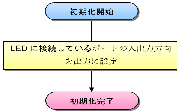
図 8.2-33 LED 初期化のフローチャート
