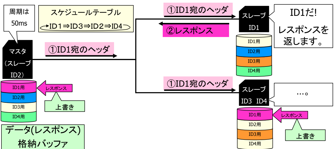
図 10.1-10 LIN 通信手順Ⅳ
