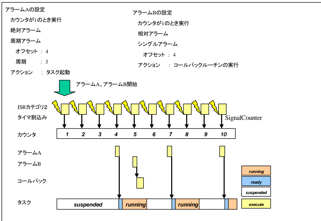
図 6.3-1 アラームの動作
