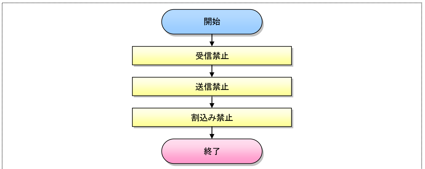
図 10.2-8. UART 送受信の禁止依存部関数 hw_lin_uart_disable フローチャート
