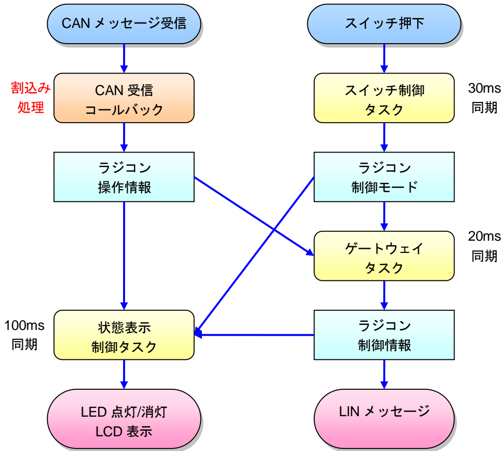
図 11.1-7 タスクと制御データの関連図
