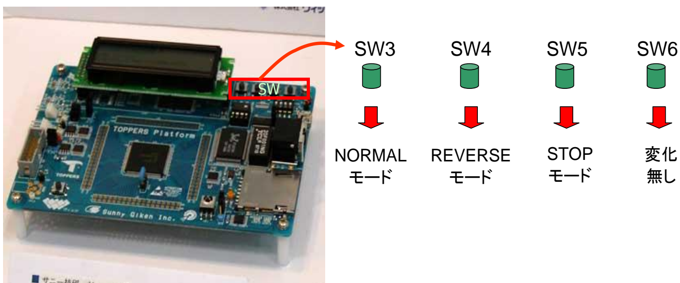
図 11.1-4 制御モード情報取得イメージ図
