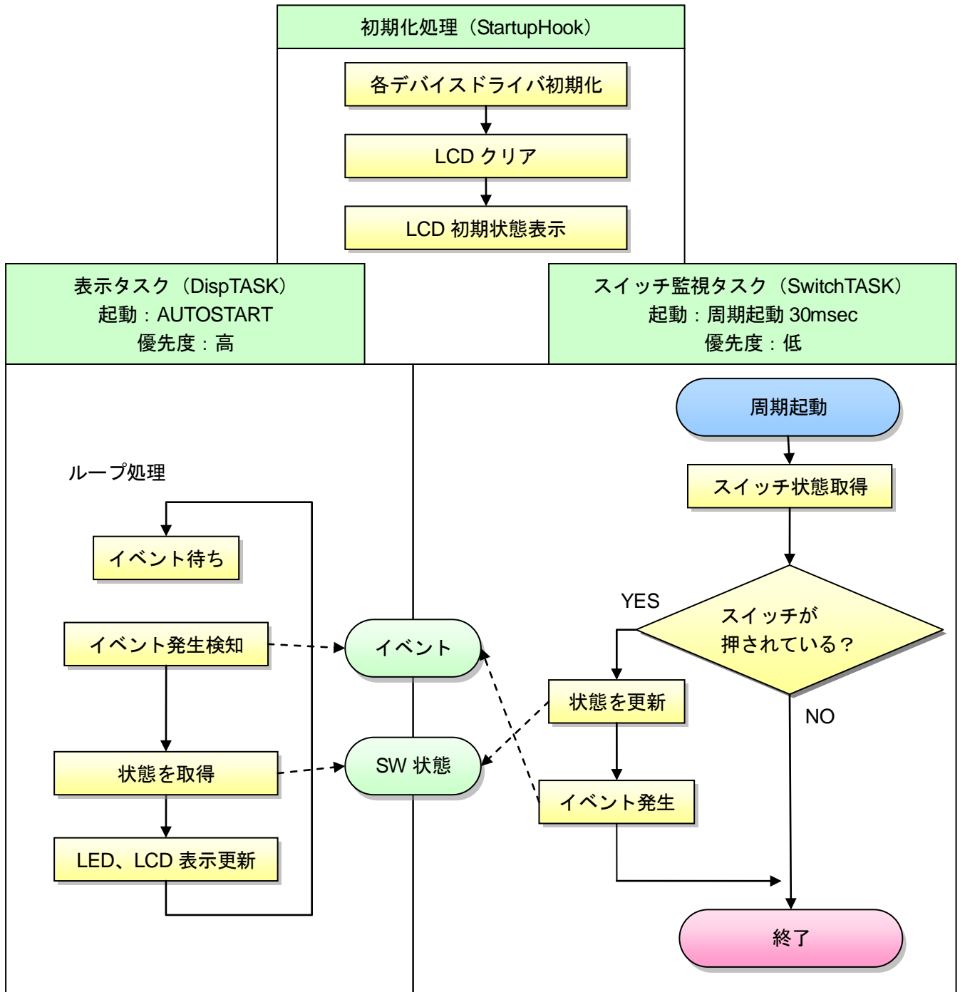
図 8.4-2 デバイスドライバアプリケーション 全体処理フロー
