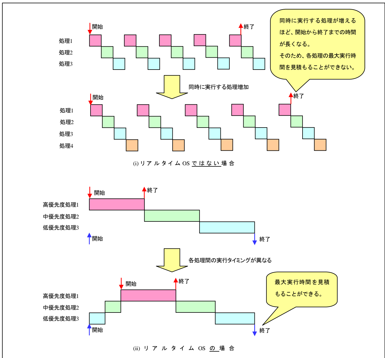
図 2.3-3 汎用 OS とリアルタイム OS の動きの違い
