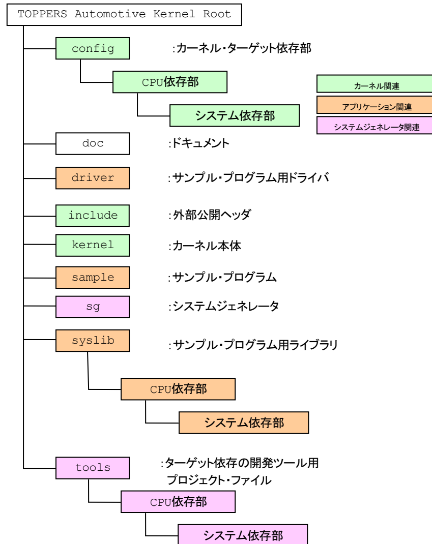
図 5.1-1 TOPPERS Automotive Kernel ディレクトリ階層
