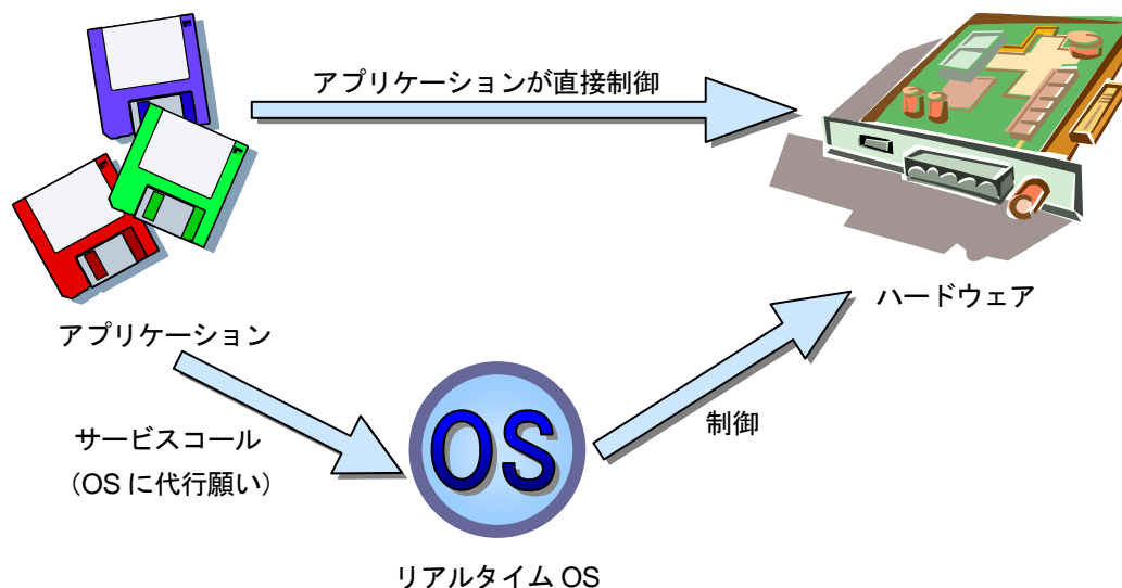
図 2.5-1 ハードウェアを制御する2つの方法
