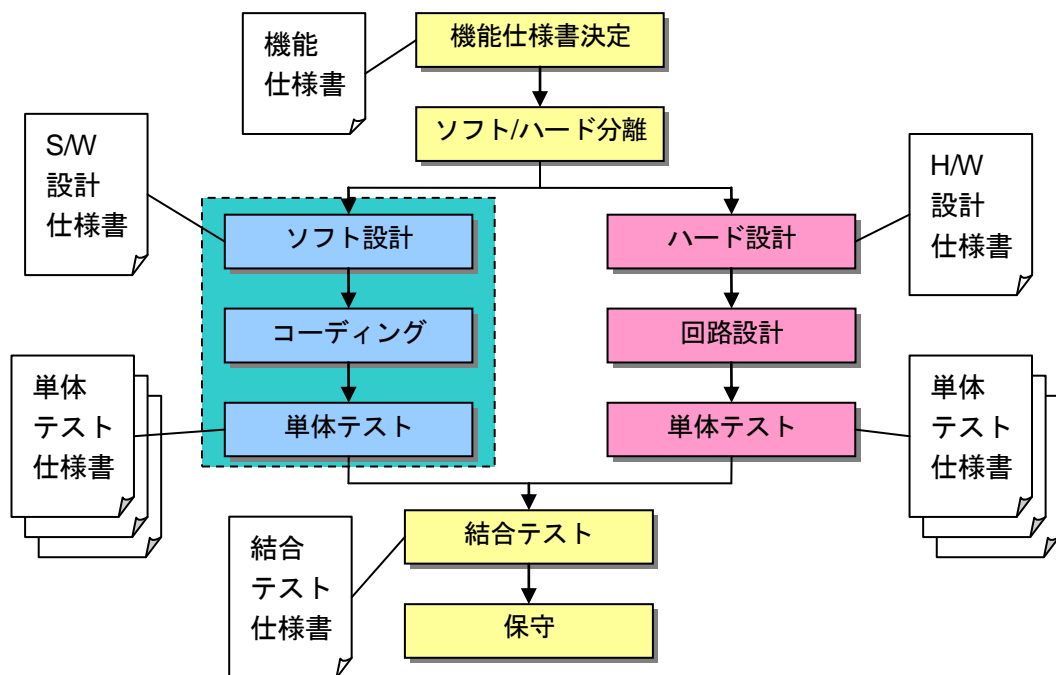
図 4.1-1 組込みシステムの開発フロー
