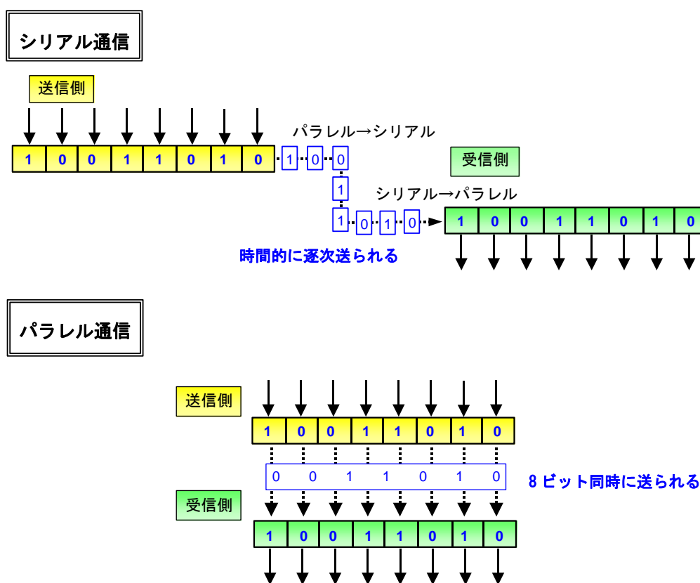
図 8.2-2 シリアル通信とパラレル通信
