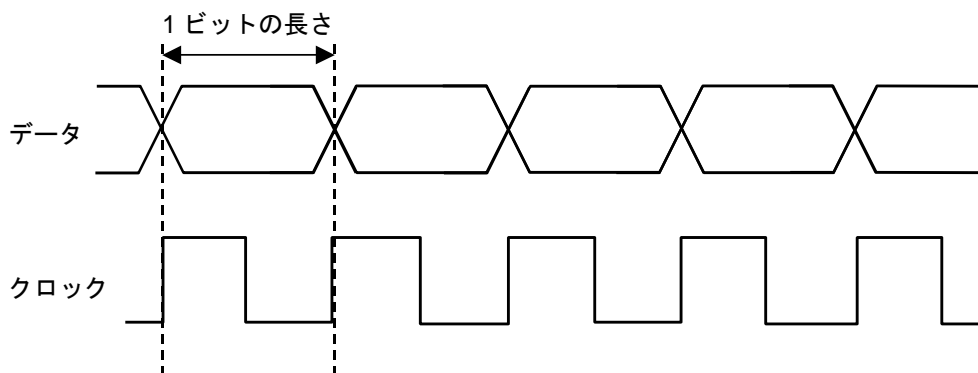
図 8.2-4 同期通信のタイムチャート
