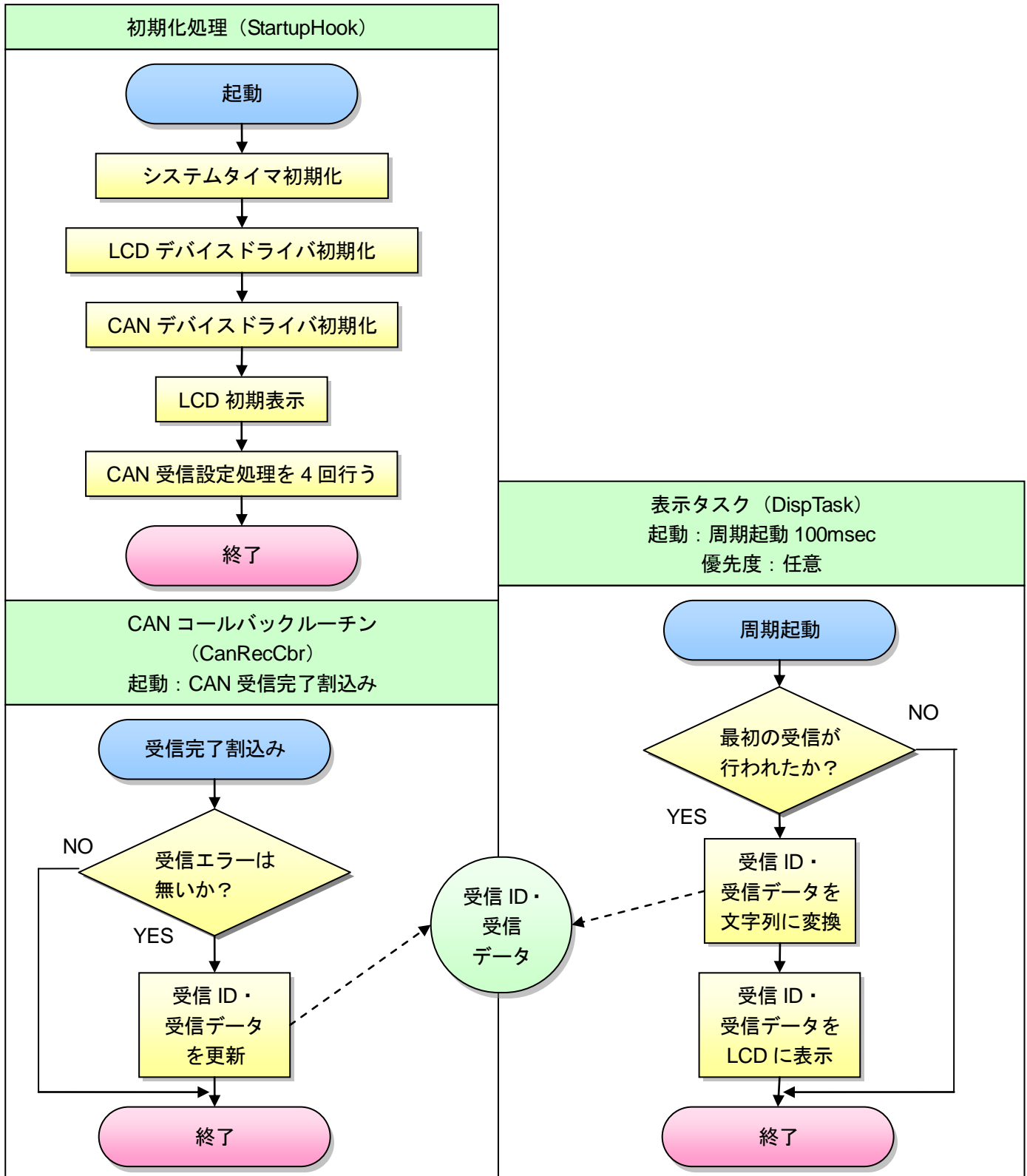
図 9.3-3 受信アプリケーション処理フロー
