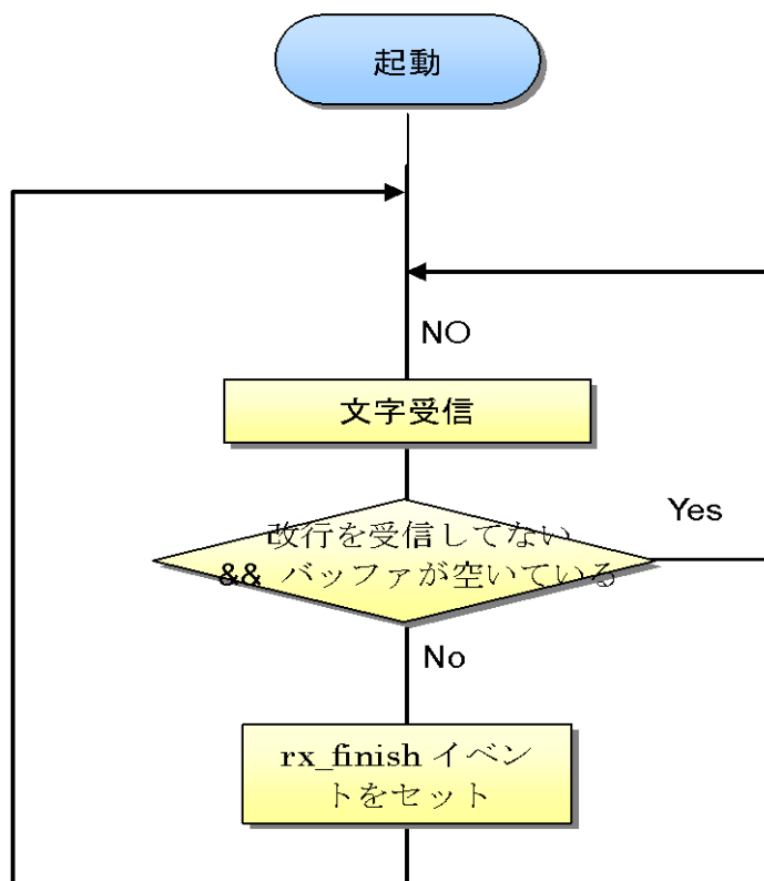
図 8.2-52 ReceiveTASK のフローチャート
