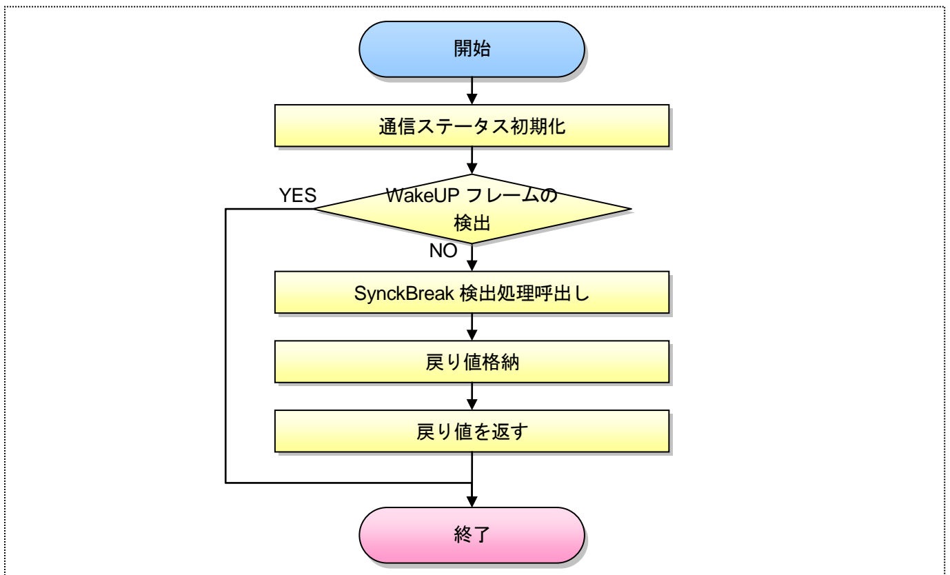
図 10.2-19. Synch Break 開始処理 sts_sb フローチャート
