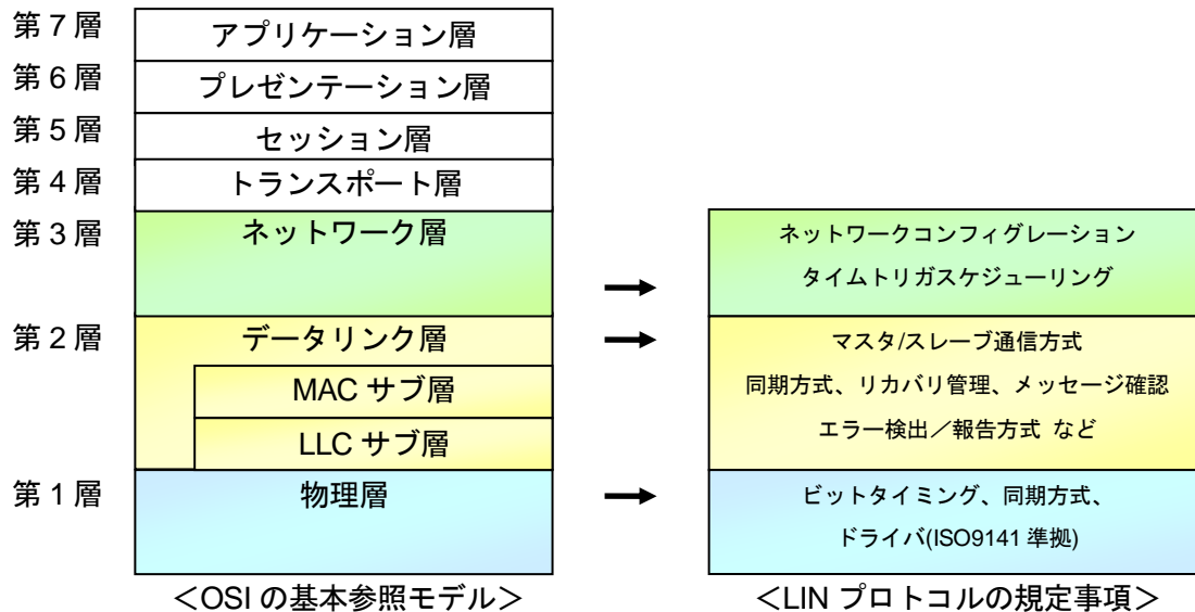
図 10.1-2 LIN における OSI 参照モデル
