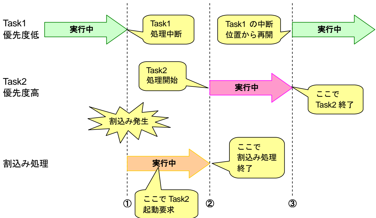
図 2.7-3 OS ありの環境での割込み処理一例
