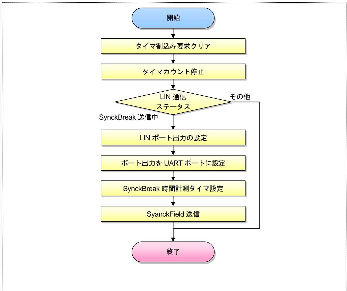
図 10.2-18. Synch Break 計測タイマ int_lin_timer フローチャート
