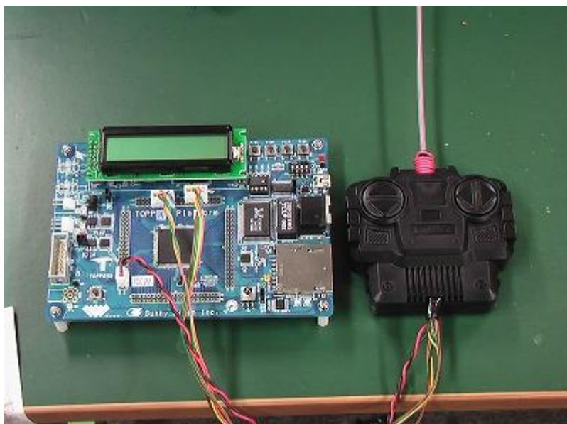
図 13.9-1 リモコン完成図
