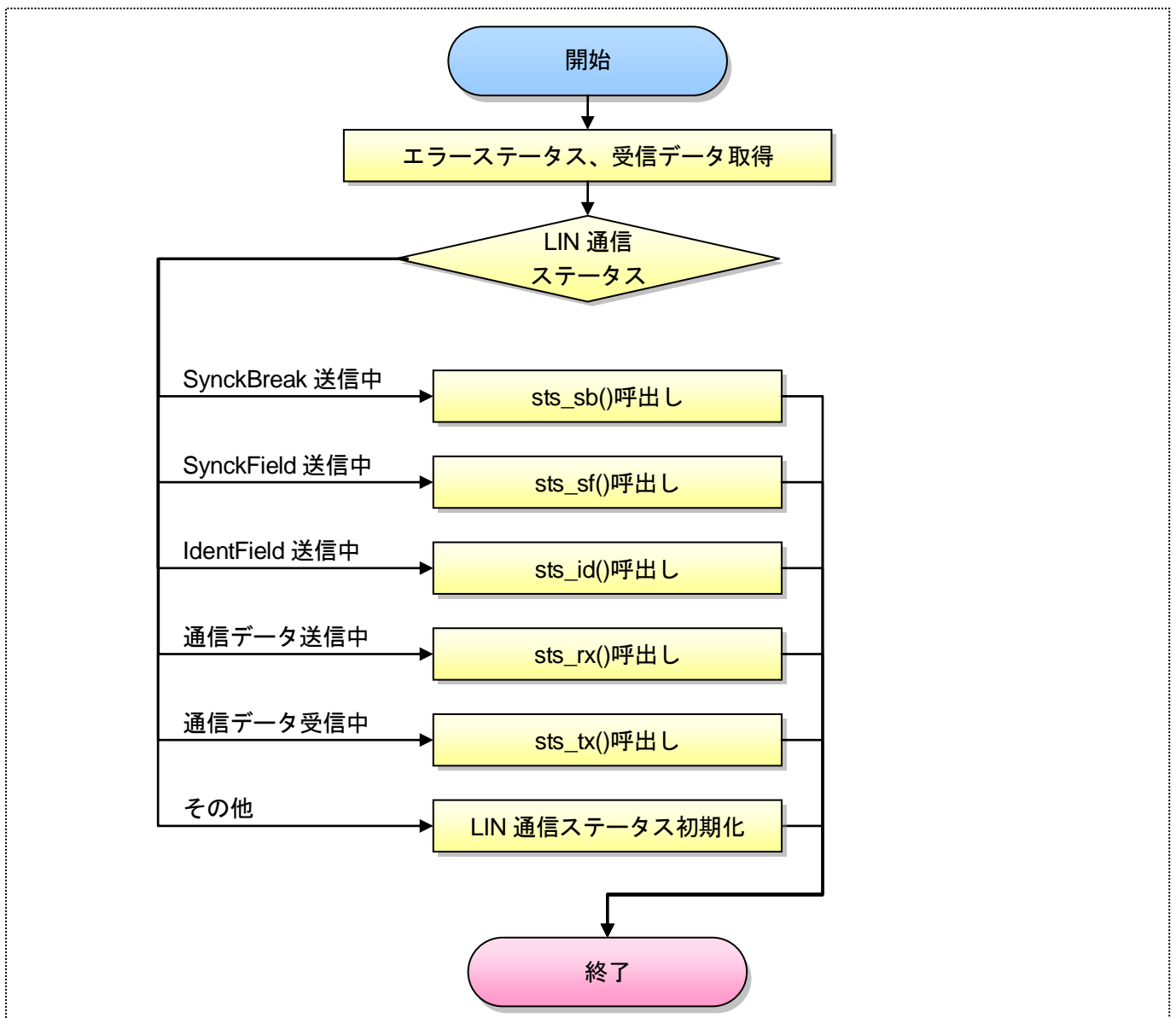
図 10.2-17. UART 受信割込み処理 lin_rx フローチャート
