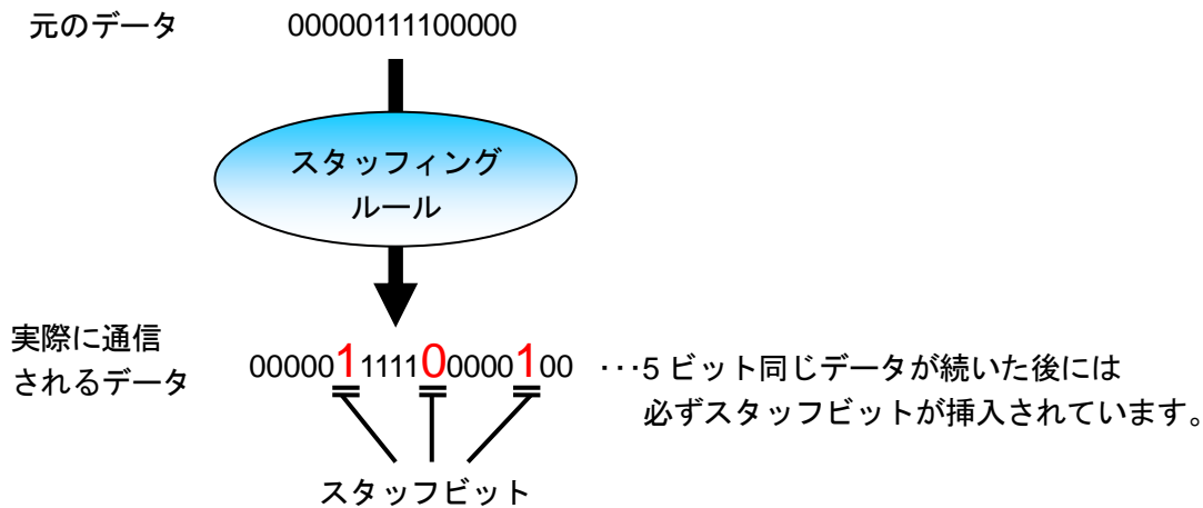
図 9.1-3 スタッフィングルール
