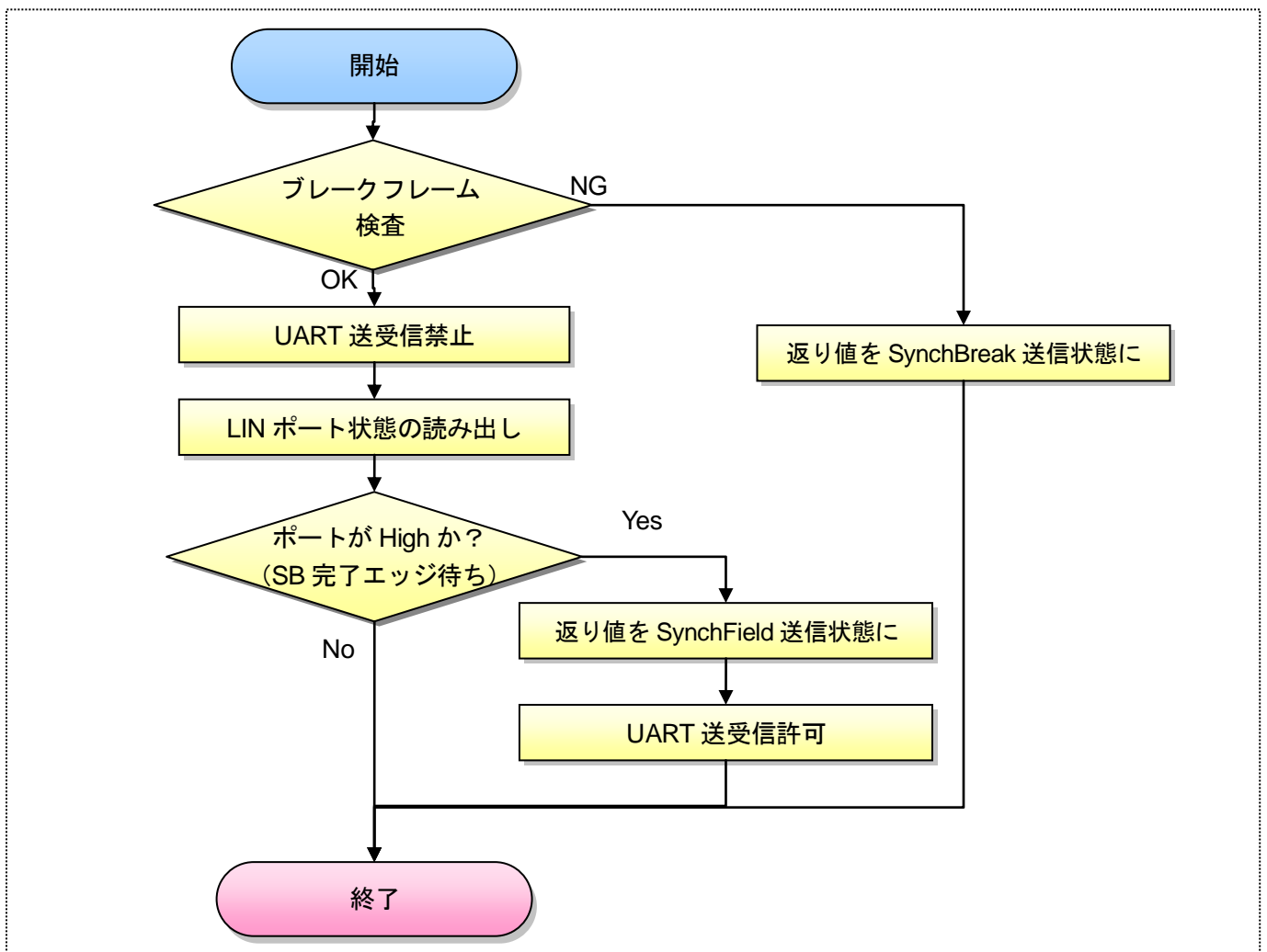
図 10.2-24. Synch Break 終了処理/エラー処理 err_proc フローチャート
