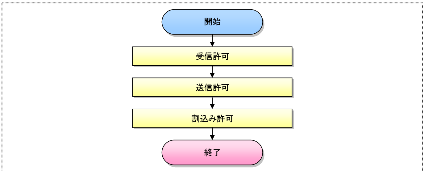
図 10.2-9. UART 送受信の許可依存部関数 hw_lin_uart_enable フローチャート
