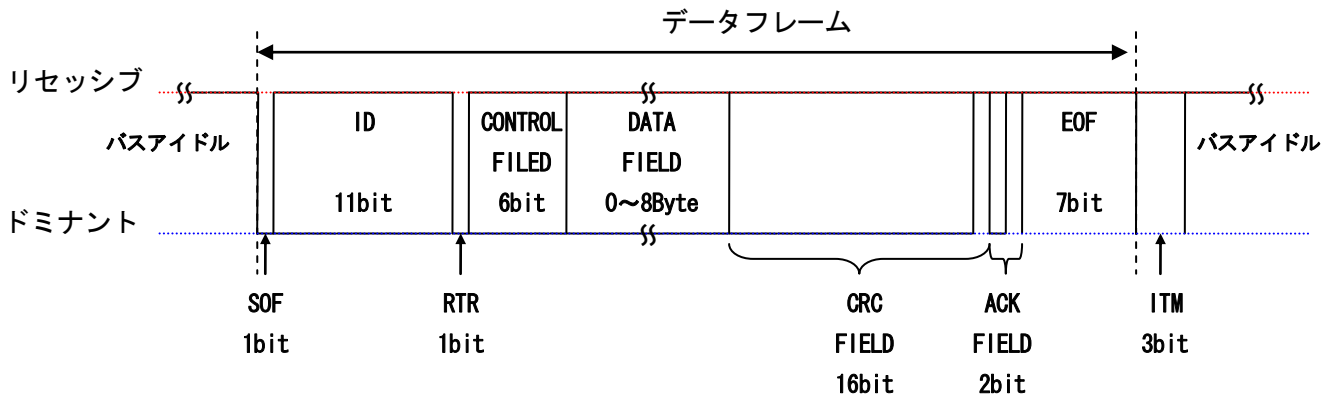
図 9.1-6 データフレーム（標準フォーマット）
