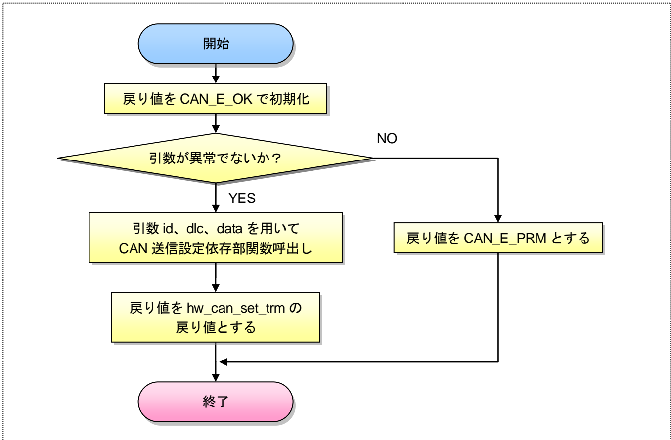
図 9.2-9 CAN 送信設定 API CanSetTrm フローチャート
