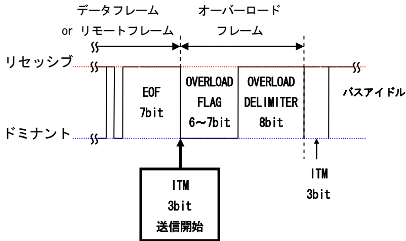
図 9.1-9 オーバーロードフレーム
