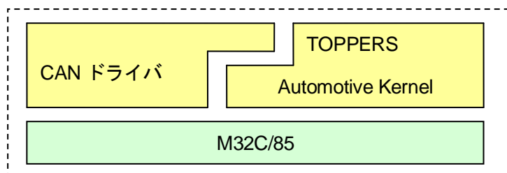
図 9.2-1 CAN デバイスドライバ構成
