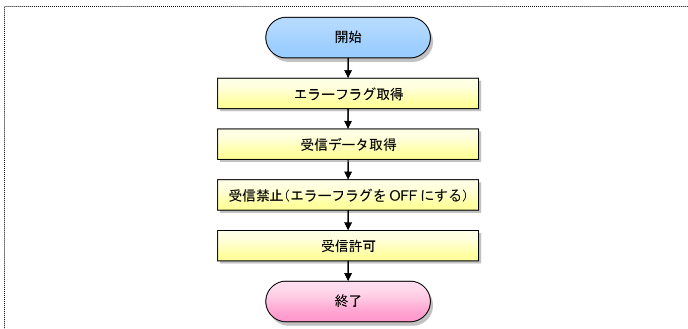
図 10.2-6. LIN データ取得依存部関数 hw_lin_uart_rx フローチャート
