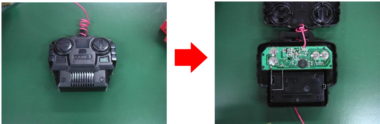
図 13.2-1 ラジコン基板取り出し
