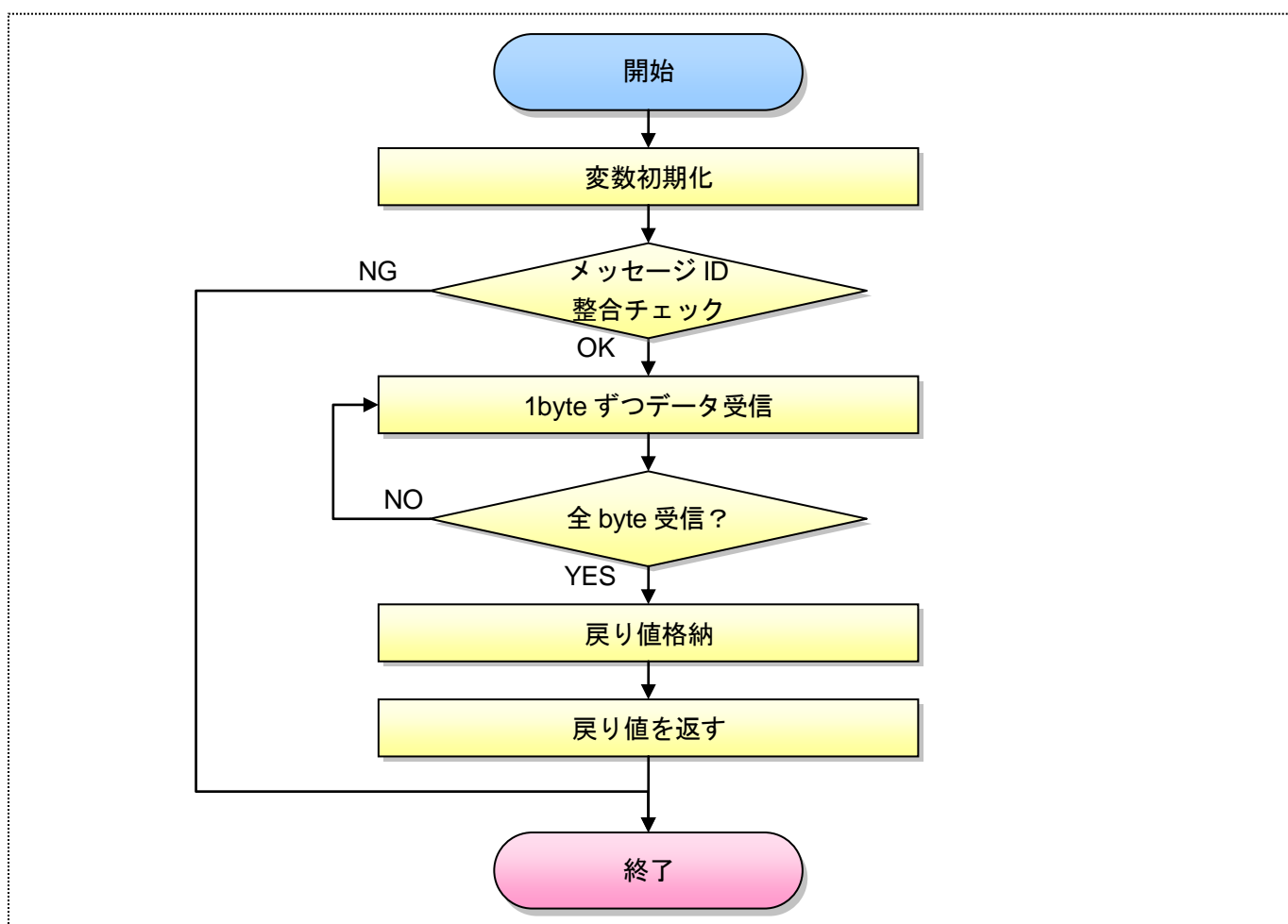
図 10.2-26. LIN データ受信処理 API LinRcvDat フローチャート
