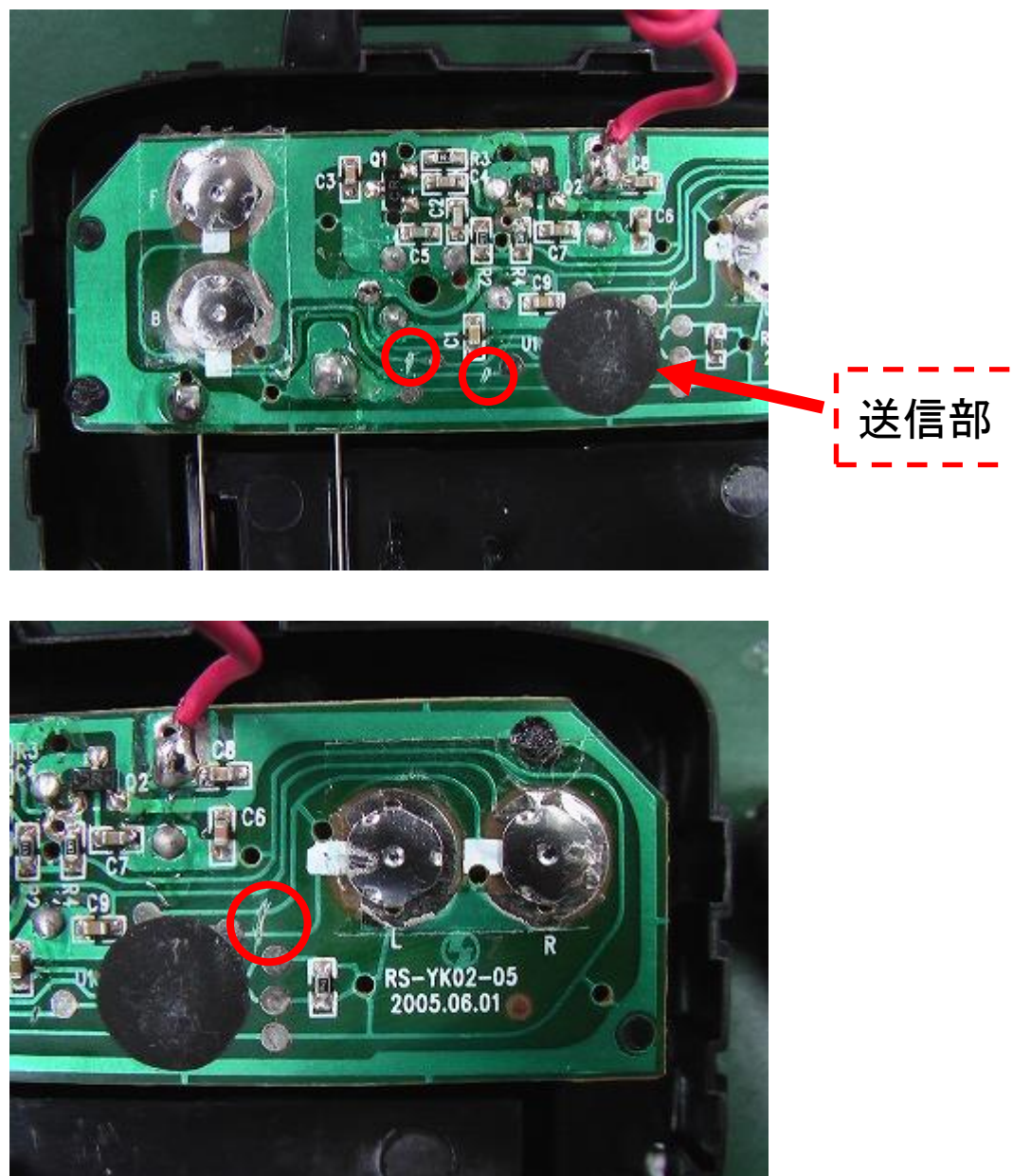
図 13.3-1 リモコン基板パターンカット
