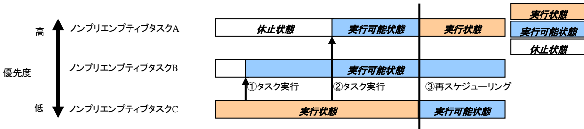
図 3.4-10 ノンプリエンティブ の例
