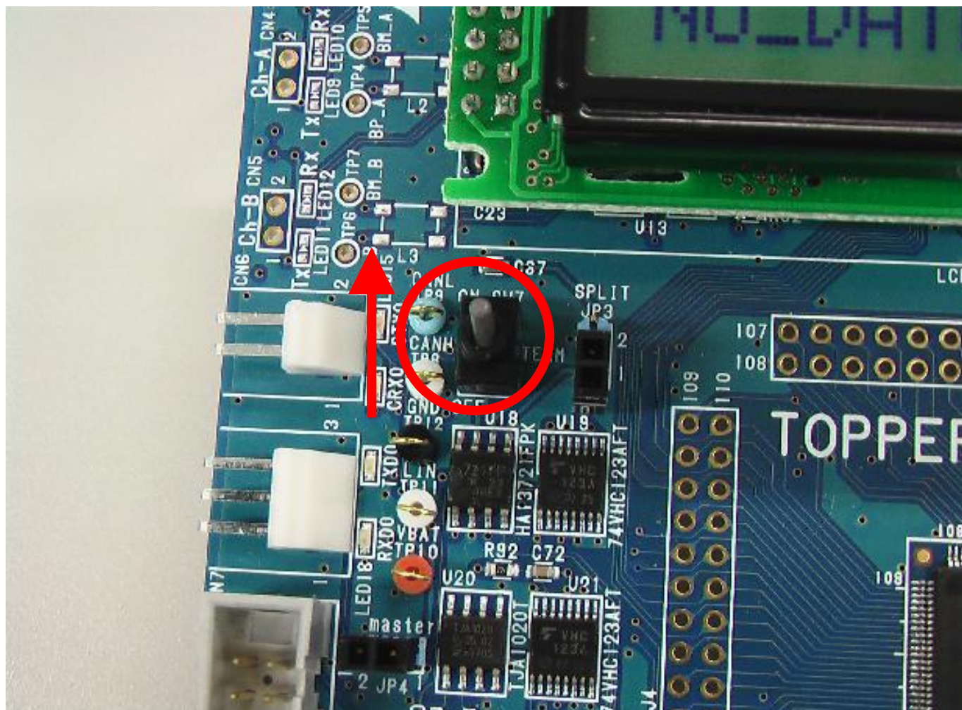
図 9.3-5 CAN 通信スイッチ設定
