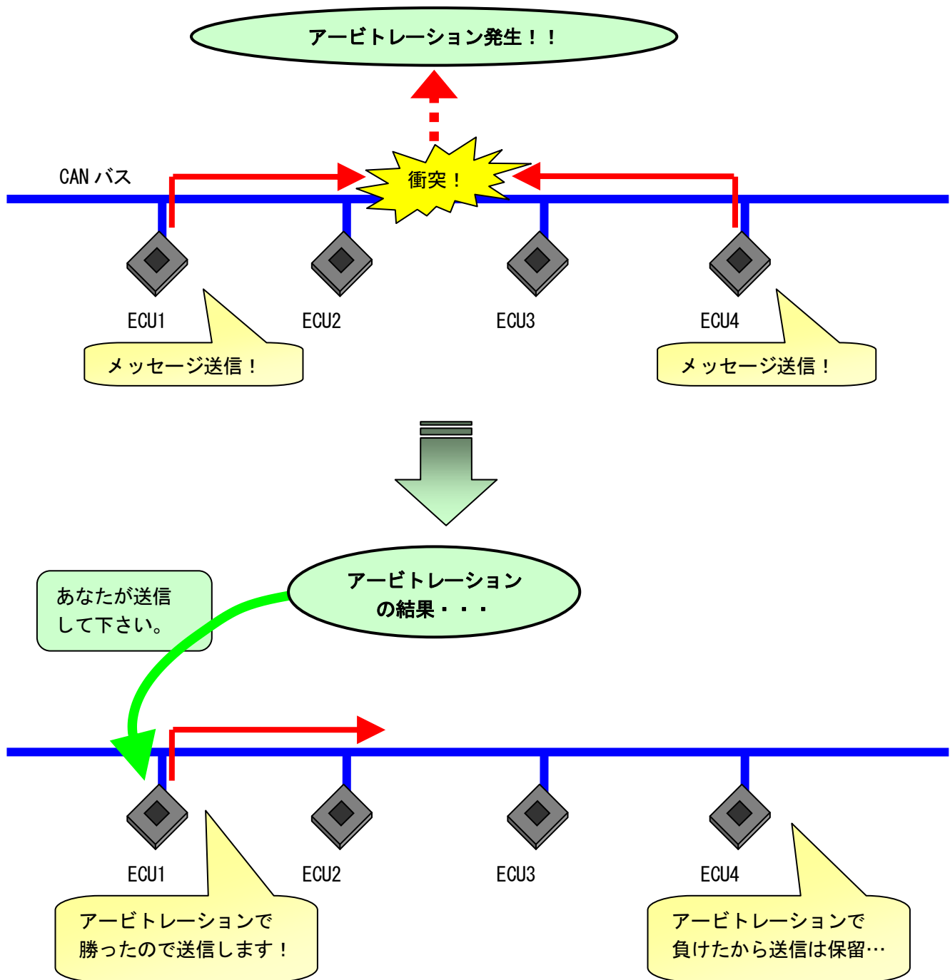
図 9.1-5 アービトレーション
