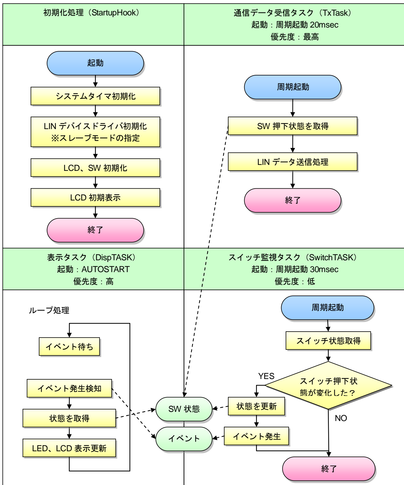
図 10.3-9 LIN デバイスドライバ動作確認アプリ仕様
