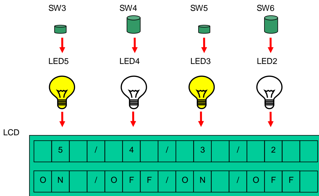
図 8.4-1 デバイスドライバアプリケーション システム概要
