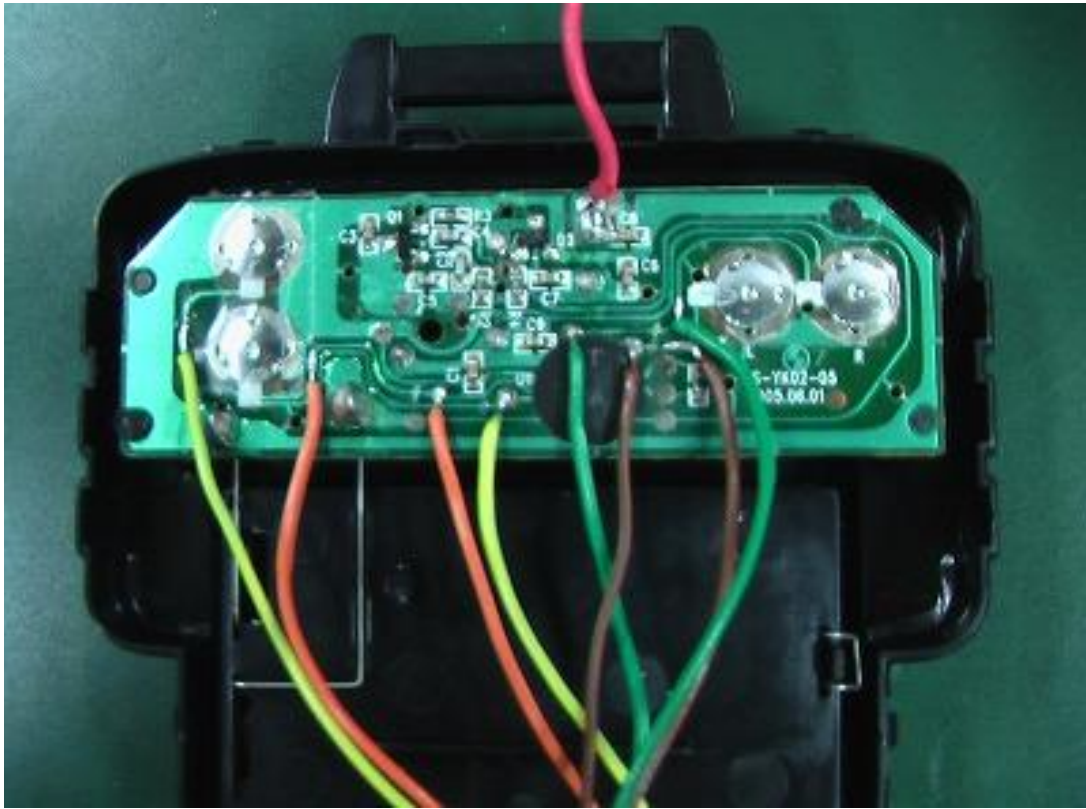
図 13.4-1 ケーブルハンダ付け
