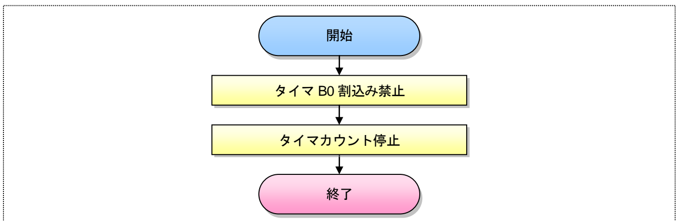
図 10.2-13. 時間計測用タイマの停止依存部関数 hw_lin_timer_stop フローチャート
