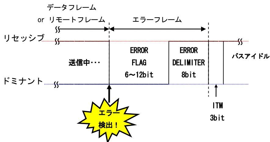
図 9.1-10 エラーフレーム
