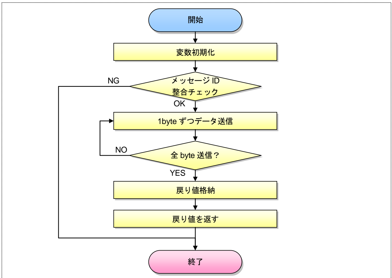
図 10.2-27. LIN データ送信処理 API LinSndDat フローチャート
