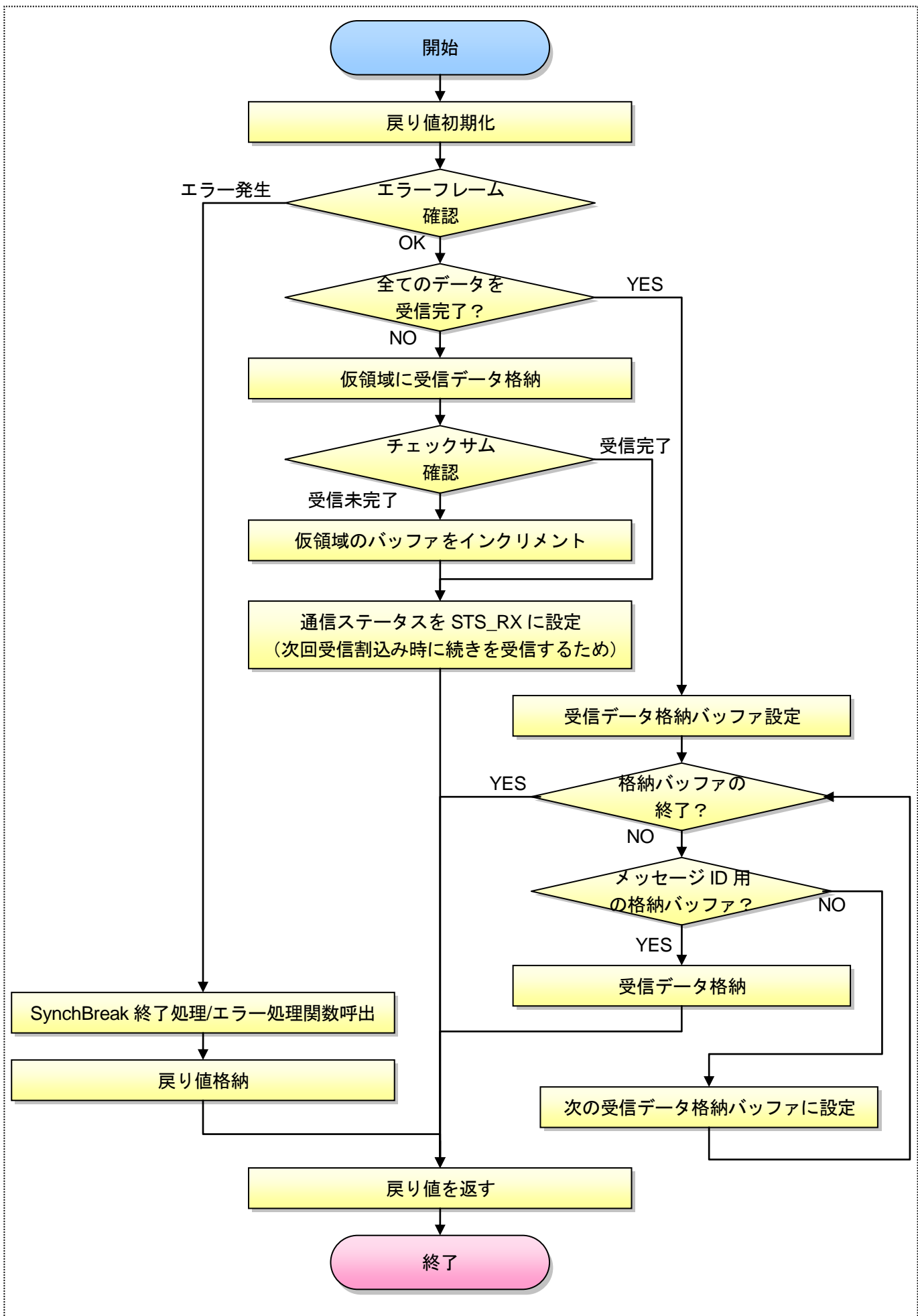
図 10.2-22. UART データ受信処理 sts_rx フローチャート
