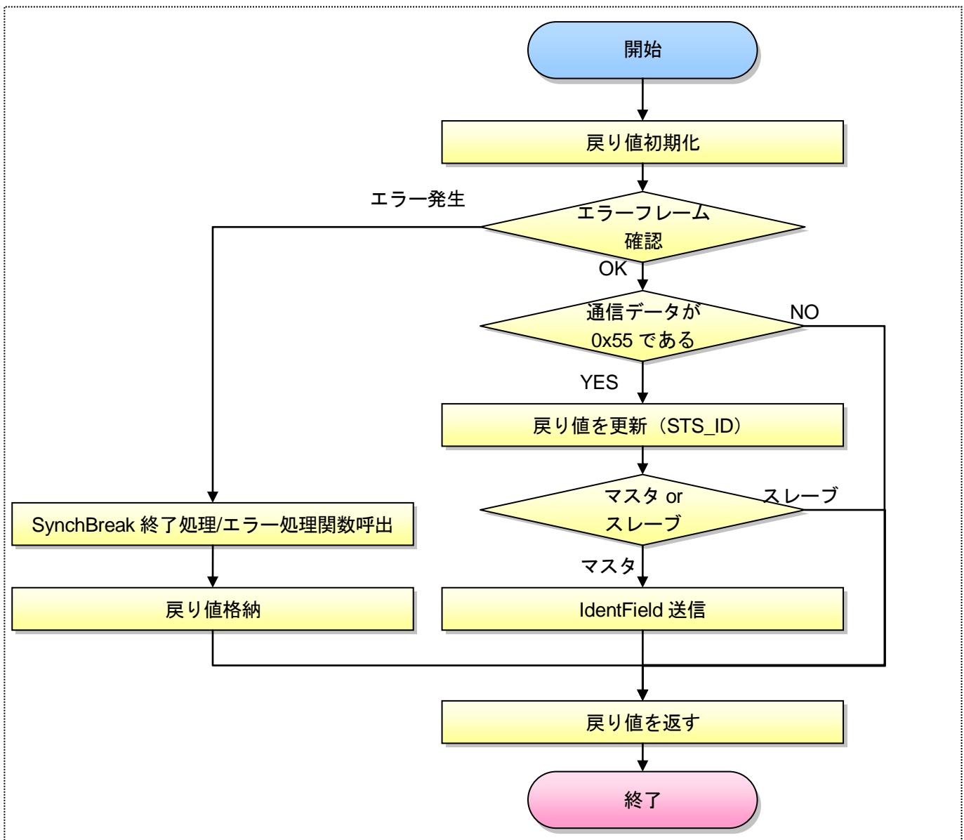
図 10.2-20. Synch Field 開始処理 sts_sf フローチャート
