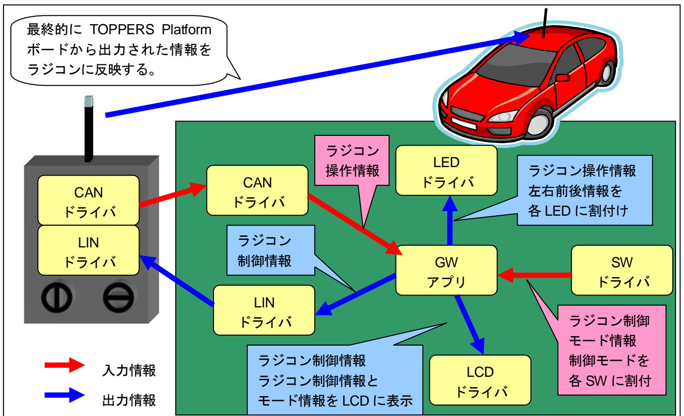
図 11.1-1 システム概要図
