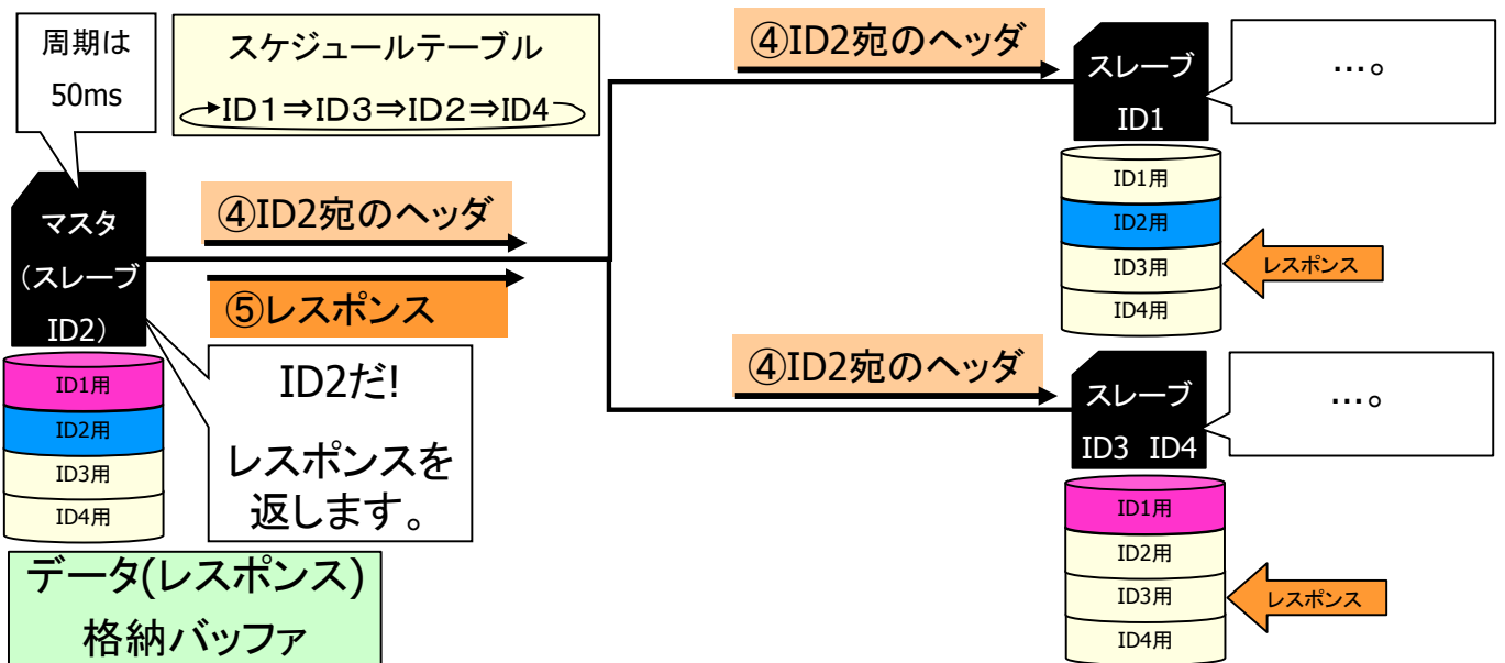
図 10.1-9 LIN 通信手順Ⅲ
