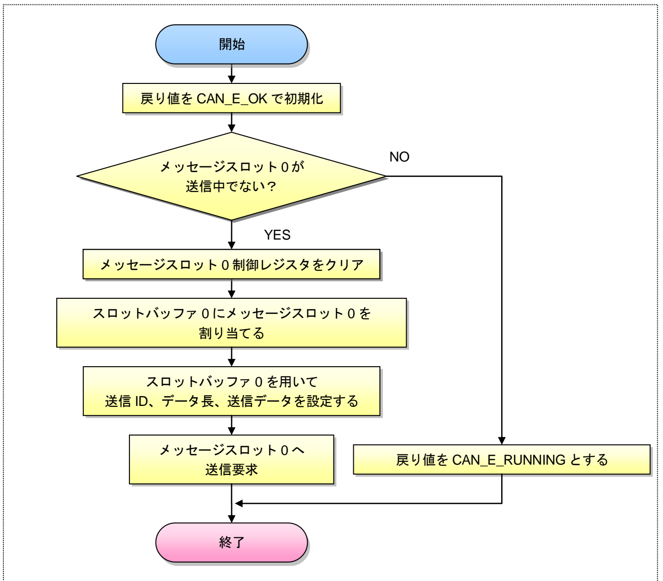
図 9.2-5 CAN 送信設定依存部関数 hw_can_set_trm フローチャート
