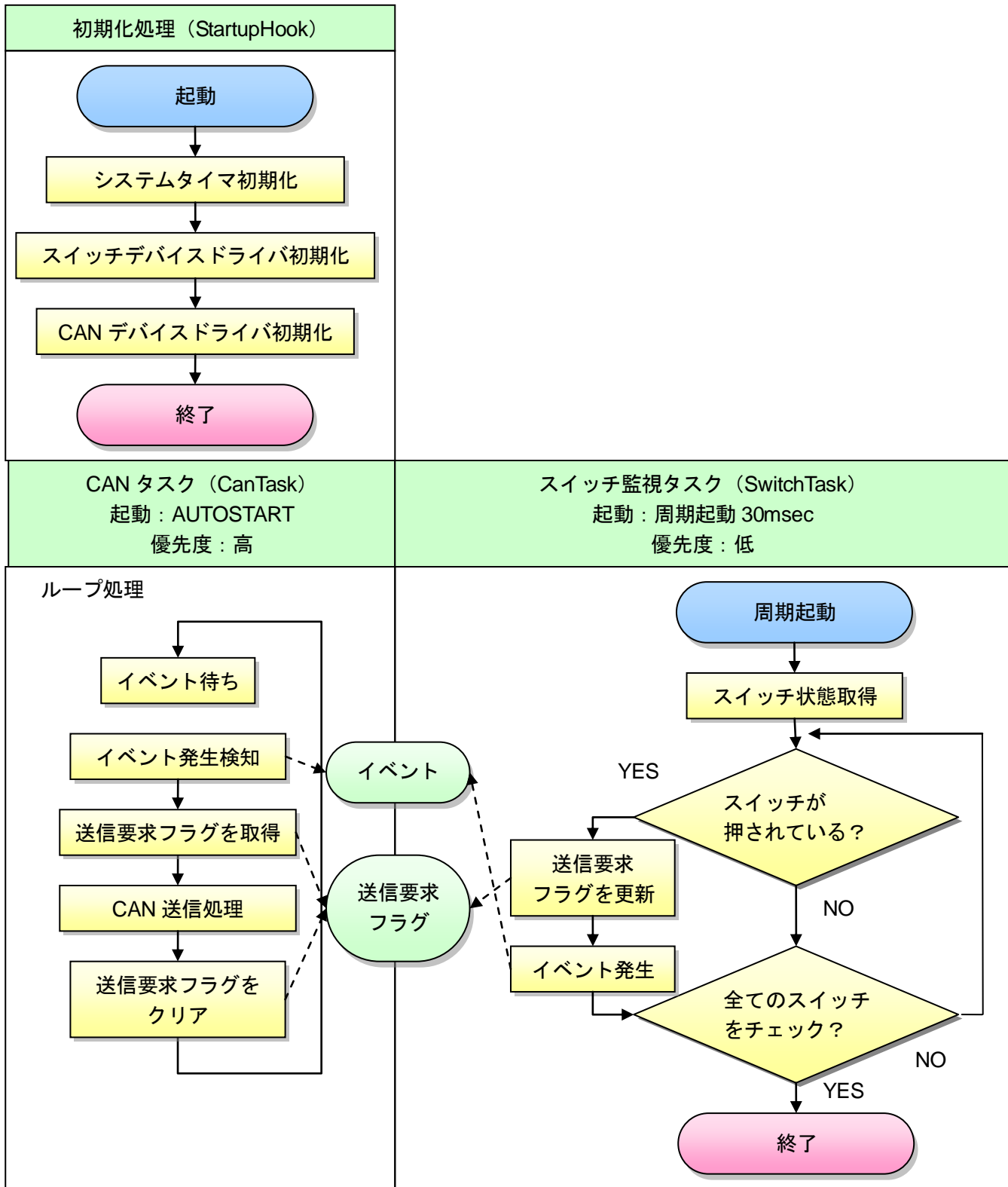
図 9.3-2 送信アプリケーション処理フロー
