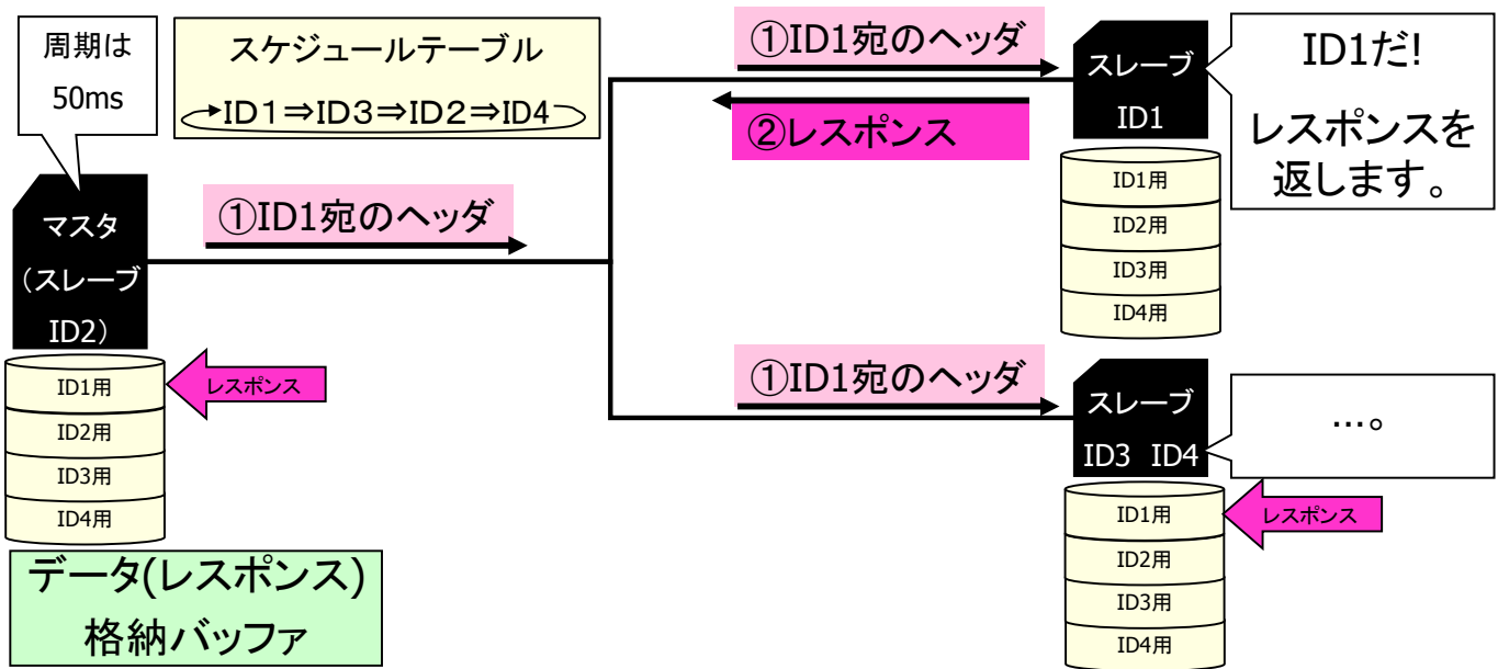
図 10.1-7 LIN 通信手順 I
