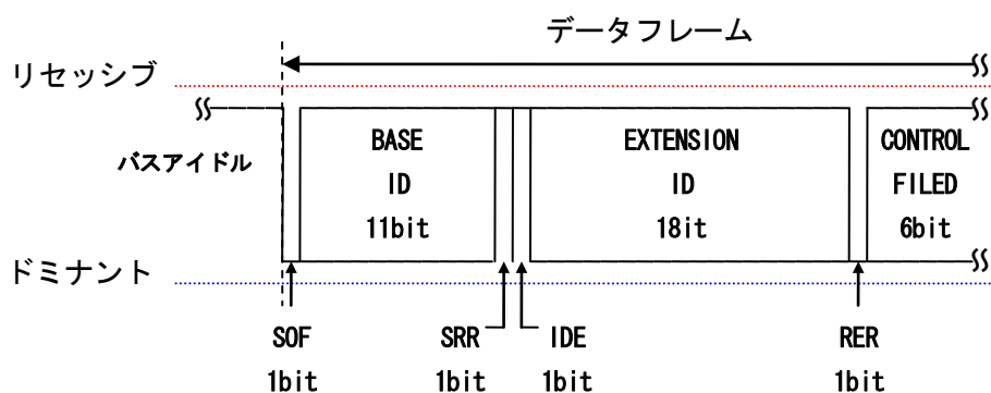
図 9.1-7 データフレーム (拡張フォーマット)
