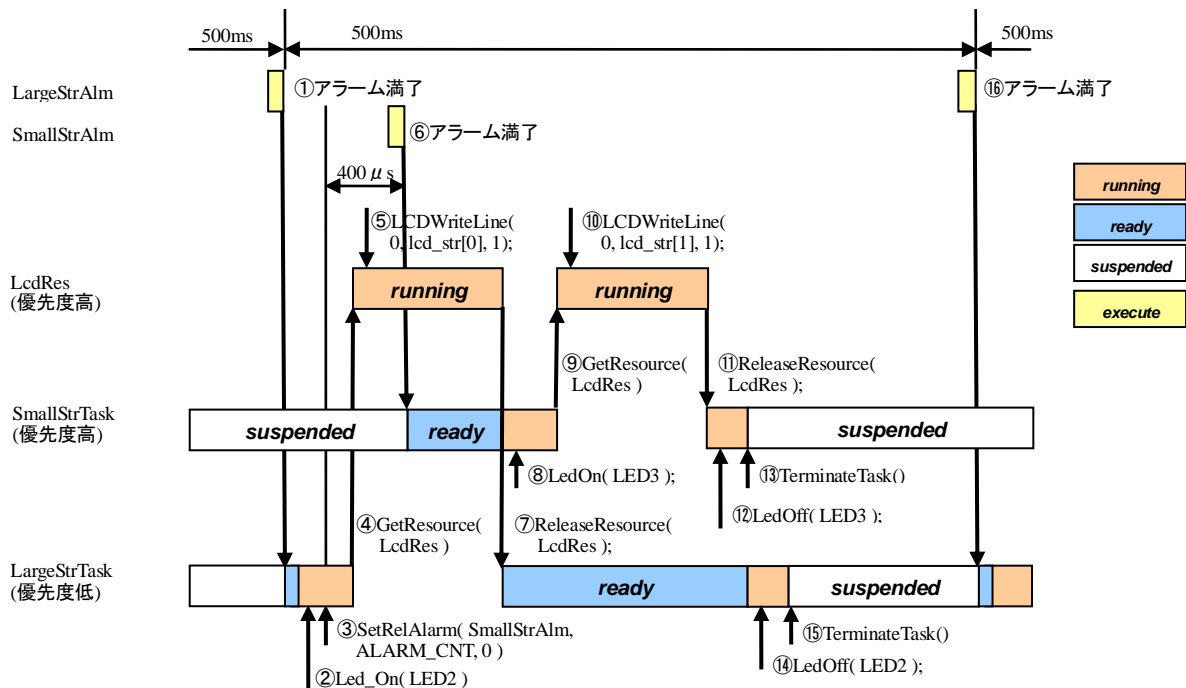
図 12.2-2 リソース使用プログラムの動作
