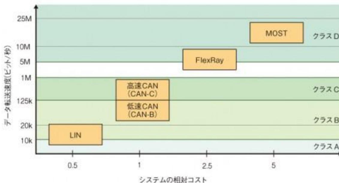
図 1.4-1 通信速度とシステムの相対コスト
