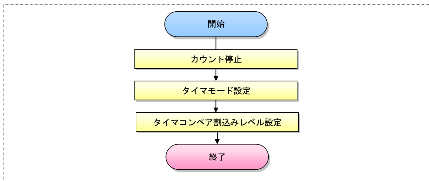
図 10.2-10. タイマ初期化依存部関数 hw_lin_timer_init フローチャート
