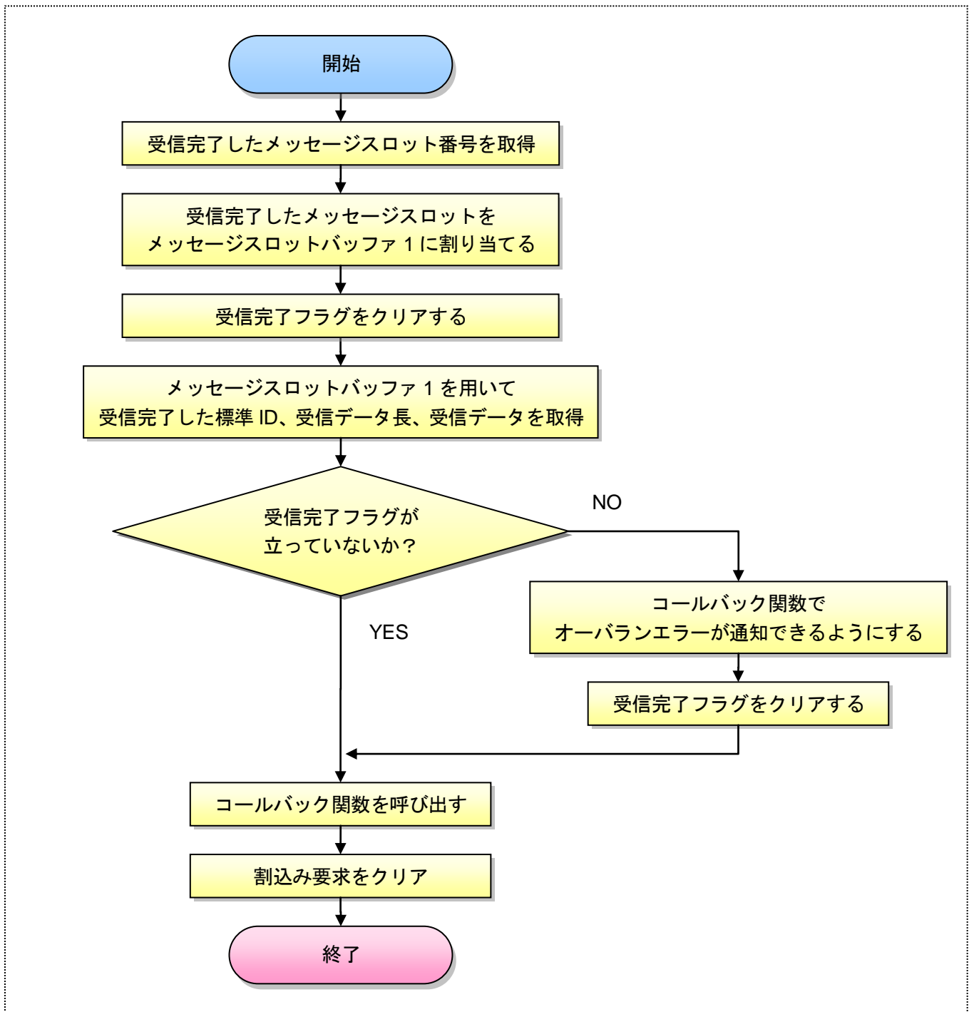
図 9.2-7 CAN 受信完了割り込み関数 hw_can_rec_int フローチャート
