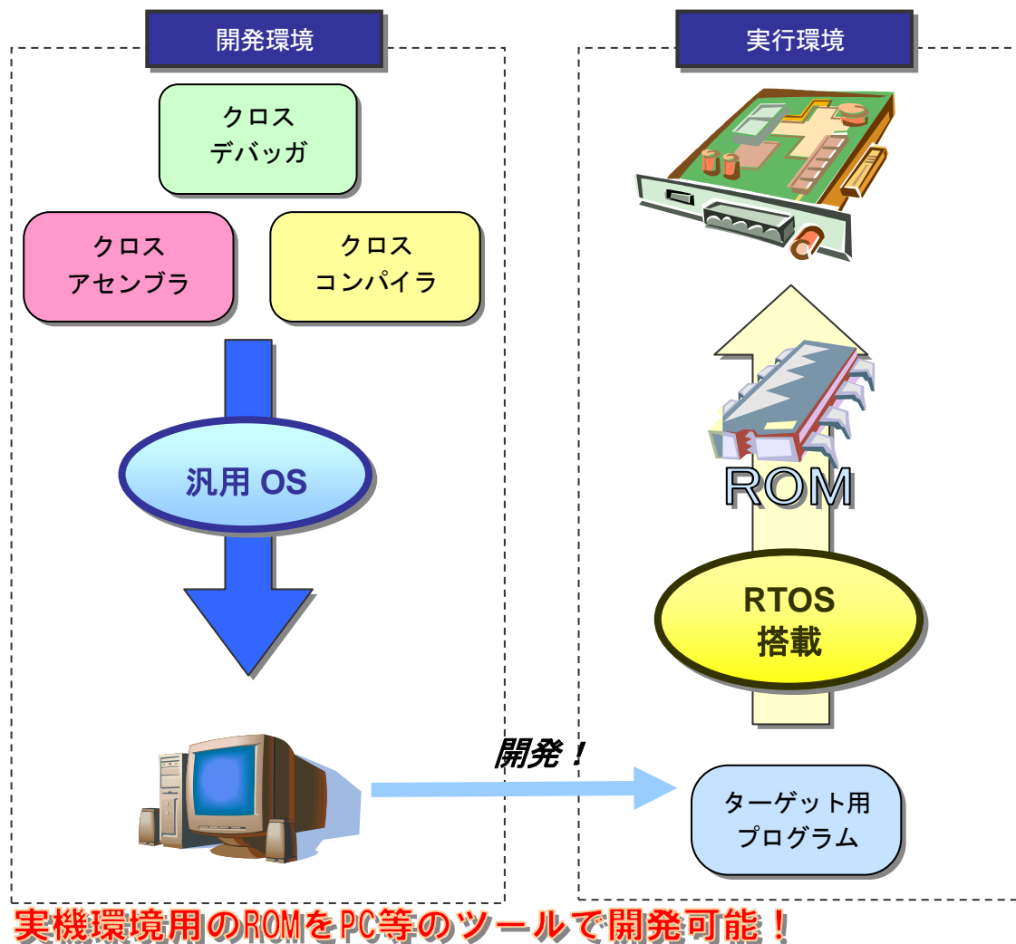
図 4.1-3 クロス開発環境
