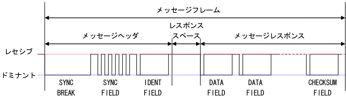
図 10.1-5 通信フレーム
