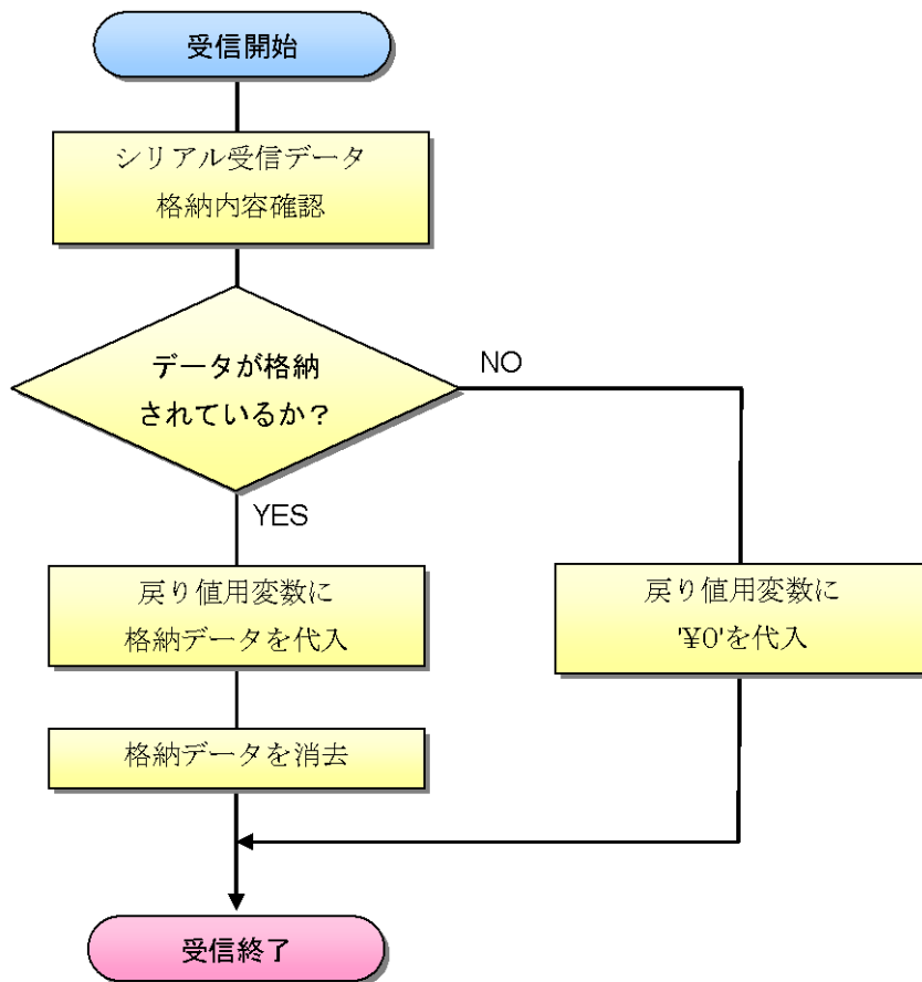
図 8.2-11 データ受信時のフローチャート
