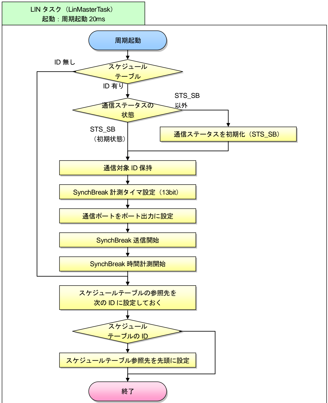
図 10.2-28. LIN マスタタスク フローチャート
