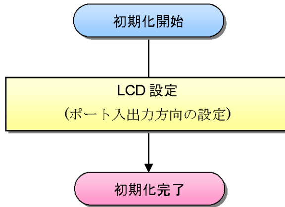
図 8.2-17 LCD 初期化のフローチャート
