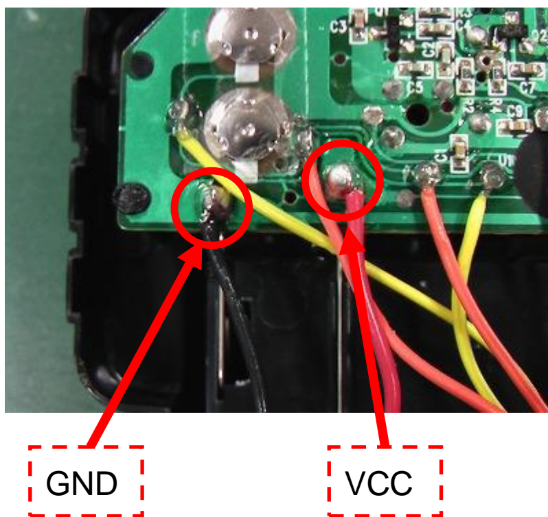
図 13.5-1 電源ケーブルハンダ付け
