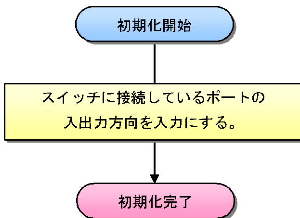
図 8.2-45 スイッチ初期化のフローチャート
