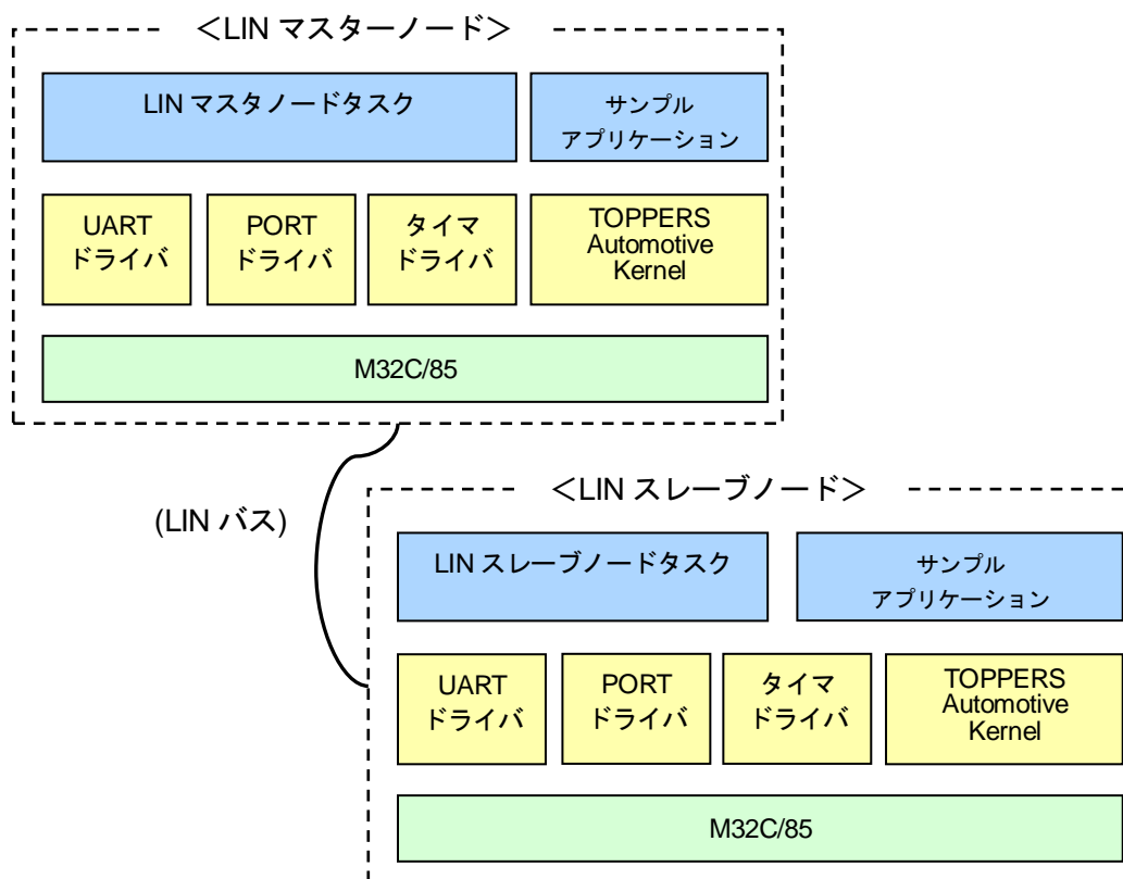
図 10.2-1. LIN ドライバ構成
