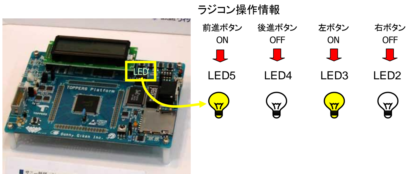
図 11.1-3 操作情報の LED 表示イメージ図
