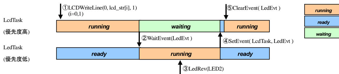
図 6.2-3 実行状態、実行可能状態、待ち状態の遷移
