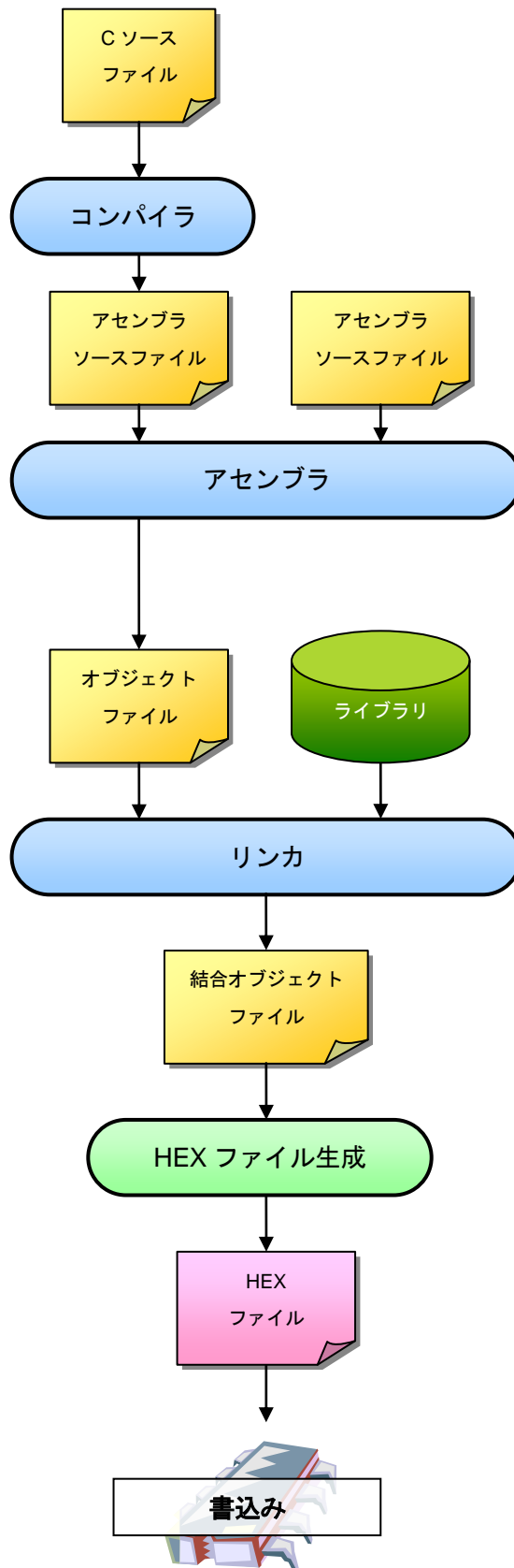
図 4.2-1 TOPPERS Automotive Kernel 未使用時の HEX ファイルができる流れ (ROM 化プログラム)
