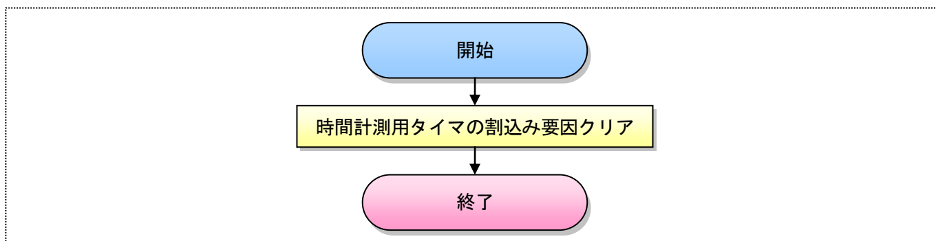
図 10.2-14. 時間計測用タイマの割込み要因クリア依存部関数 hw_lin_timer_intreq_clear フローチャート
