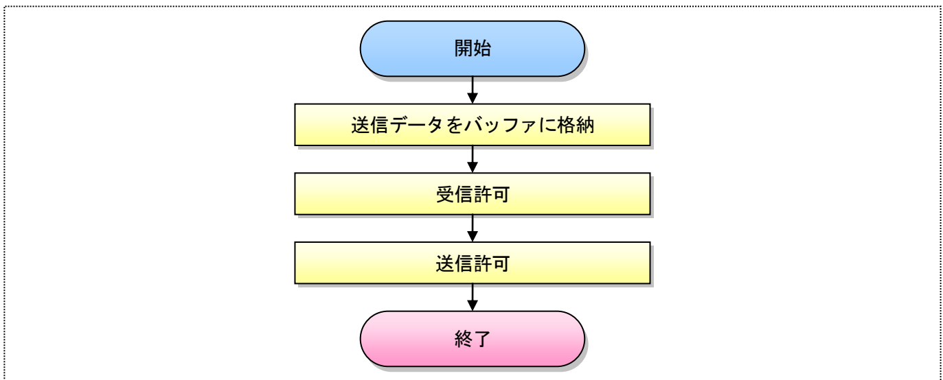
図 10.2-7. LIN データ送信依存部関数 hw_lin_uart_tx フローチャート
