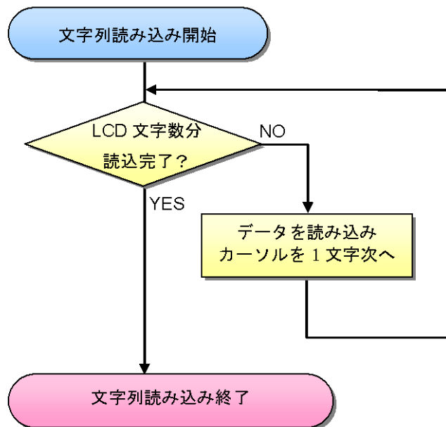
図 8.2-29 LCD データ文字列読み込みのフローチャート
