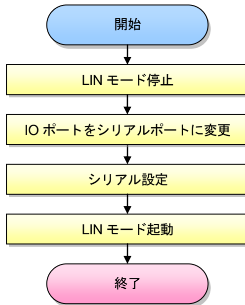
図 10.2-5. LIN ポートの UART モードへの設定依存部関数 hw_lin_uart_set_uartport フローチャート
