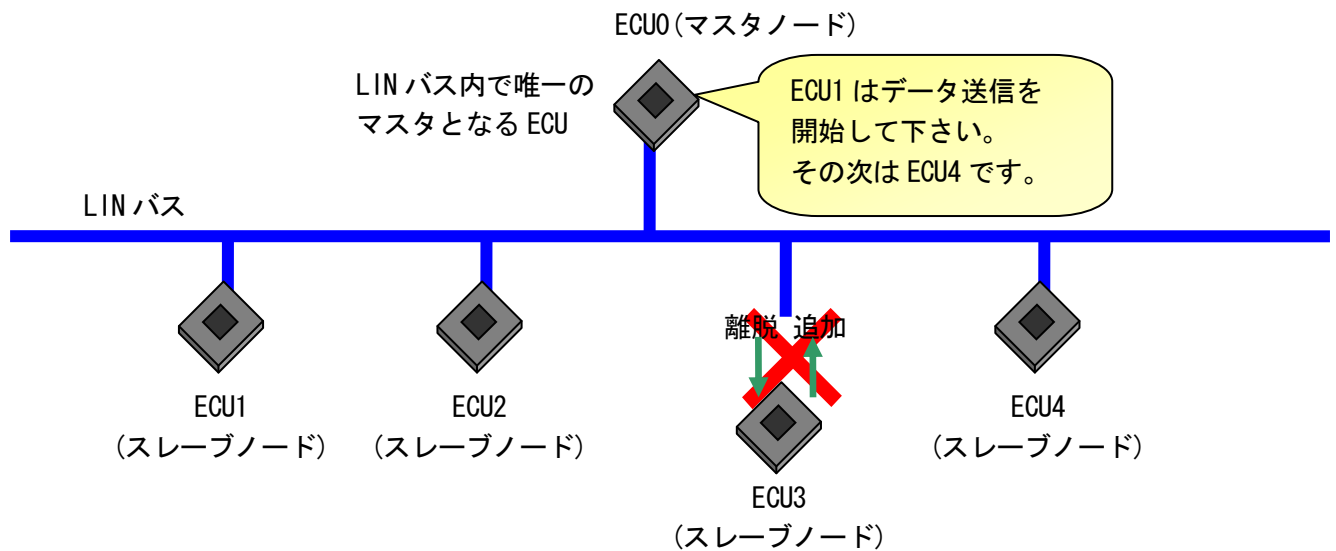
図 10.1-3 LIN バス
