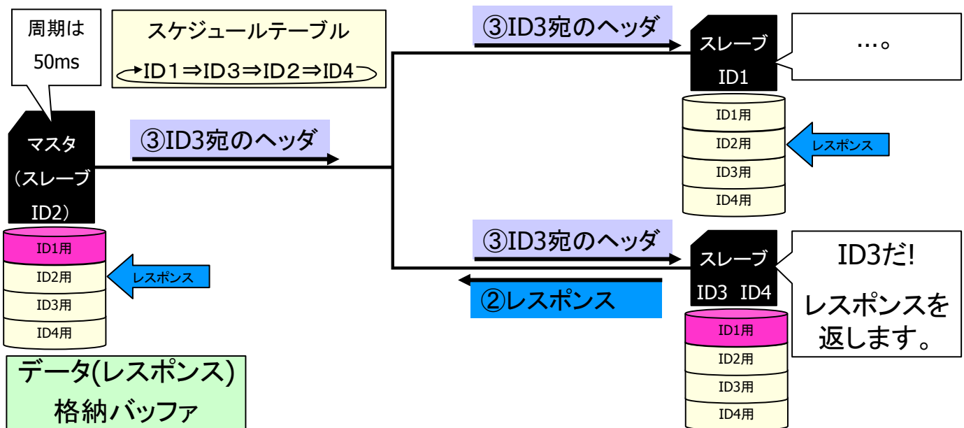
図 10.1-8 LIN 通信手順 II
