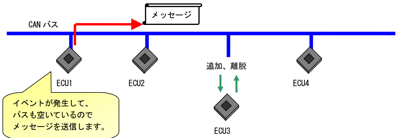
図 9.1-4 マルチマスタ方式 / イベントドリブン方式
