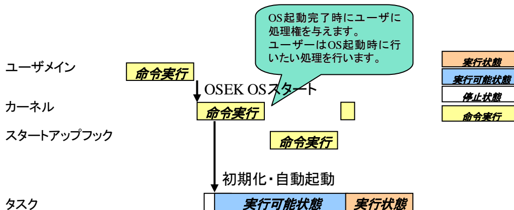
図 3.4-15 スタートアップフックの例
